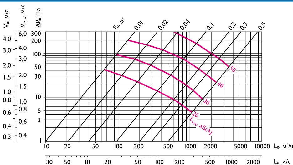
Аэродинамические и акустические характеристики решеток АМН-К, АДН-К ( \alpha_1 = \alpha_2 = 0^\circ ), АЛН-К, АБН с камерами статического давления 1КСД при подаче и удалении воздуха в помещениях
