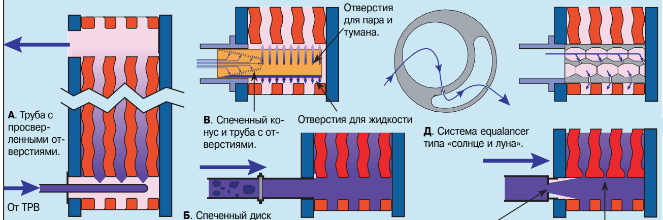
Рис. 18. Распределитель хладагента
