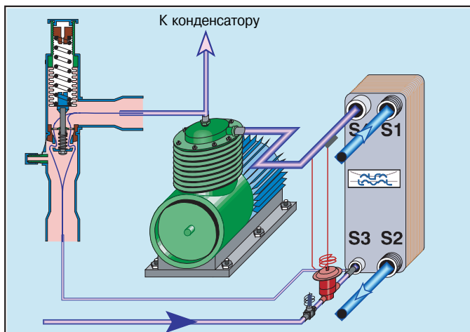
Рис. 23. Регулятор испарителя непосредственного расширения с перепуском горячего пара
