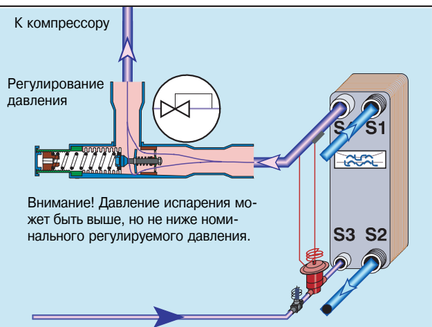
Рис. 24. Регулятор давления испарения
