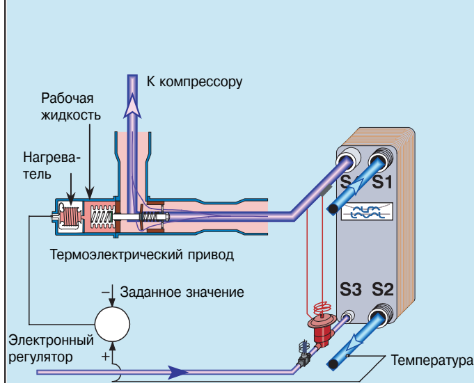
Рис. 25. Электронный регулятор давления испарения
