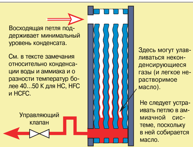
Рис. 04. Переохлаждение конденсата
