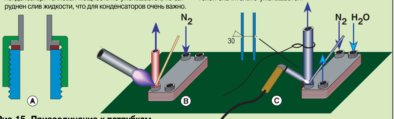
Рис. 15. Присоединение к патрубкам
