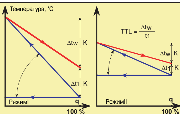
Рис. 11. Определение конечной термической длины (КТД)
