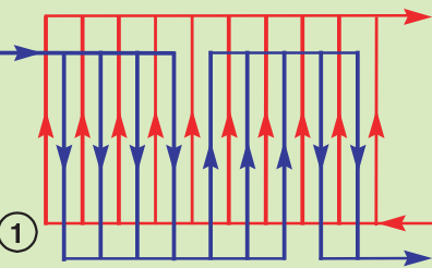
Рис. 9Б. Многоходовые схемы.
