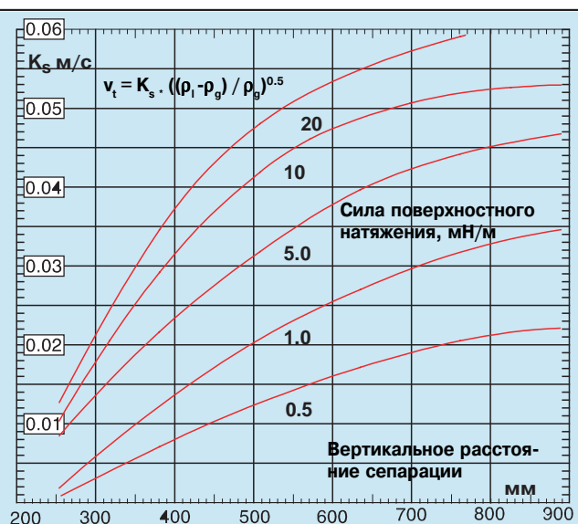
Рис. 05. Постоянная скорости Ks
