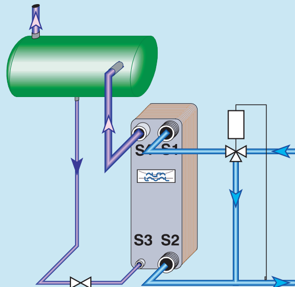
Рис. 26. Регулирование температуры в термосифонном испарителе
