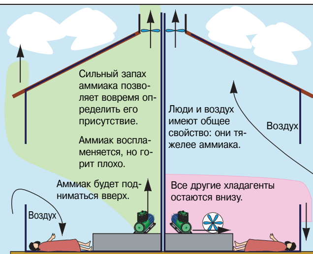
Рис. 15. Утечка хладагентов
