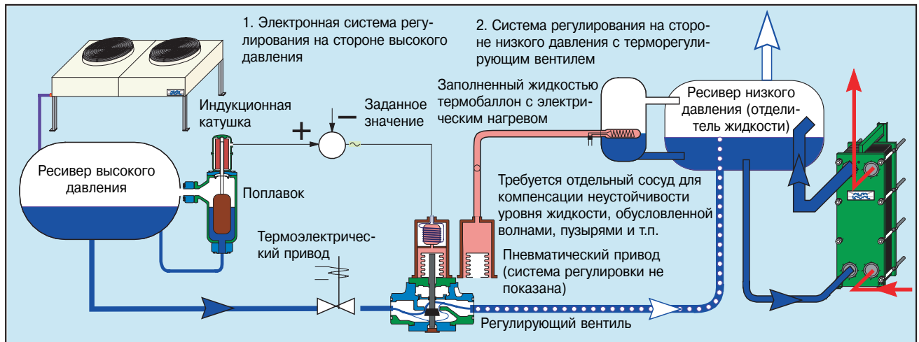
Рис. 19. Управление регулирующим вентилем в затопленном испарителе
