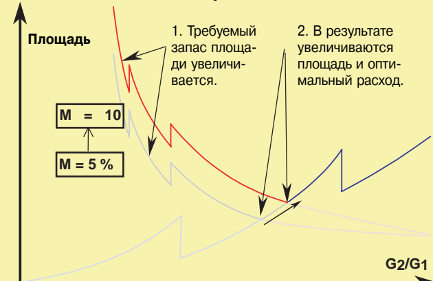
Рис. 9. Влияние увеличения запаса площади на оптимальный расход.
