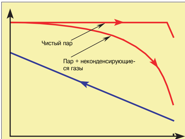
Рис. 03. Пар с неконденсирующимися газами
