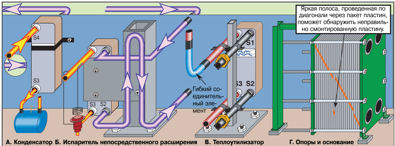
Рис. 13. Монтаж ППТО
