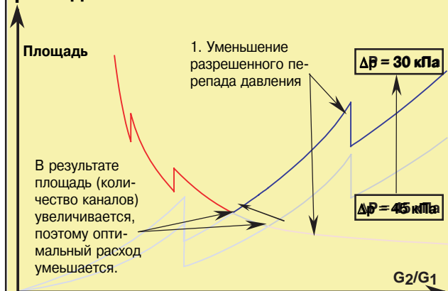
Рис. 8. Влияние уменьшения перепада давления на охлаждающей стороне на оптимальный расход.
