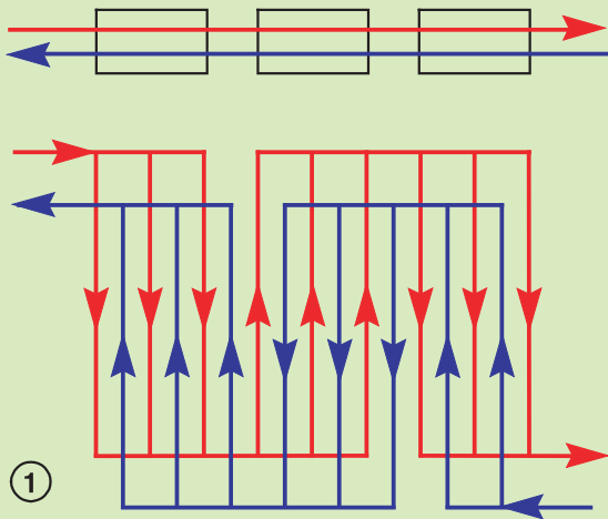
Рис. 9А. Противоток
