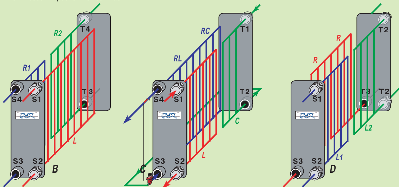
Рис. 8 В - С. Два контура / один контур
