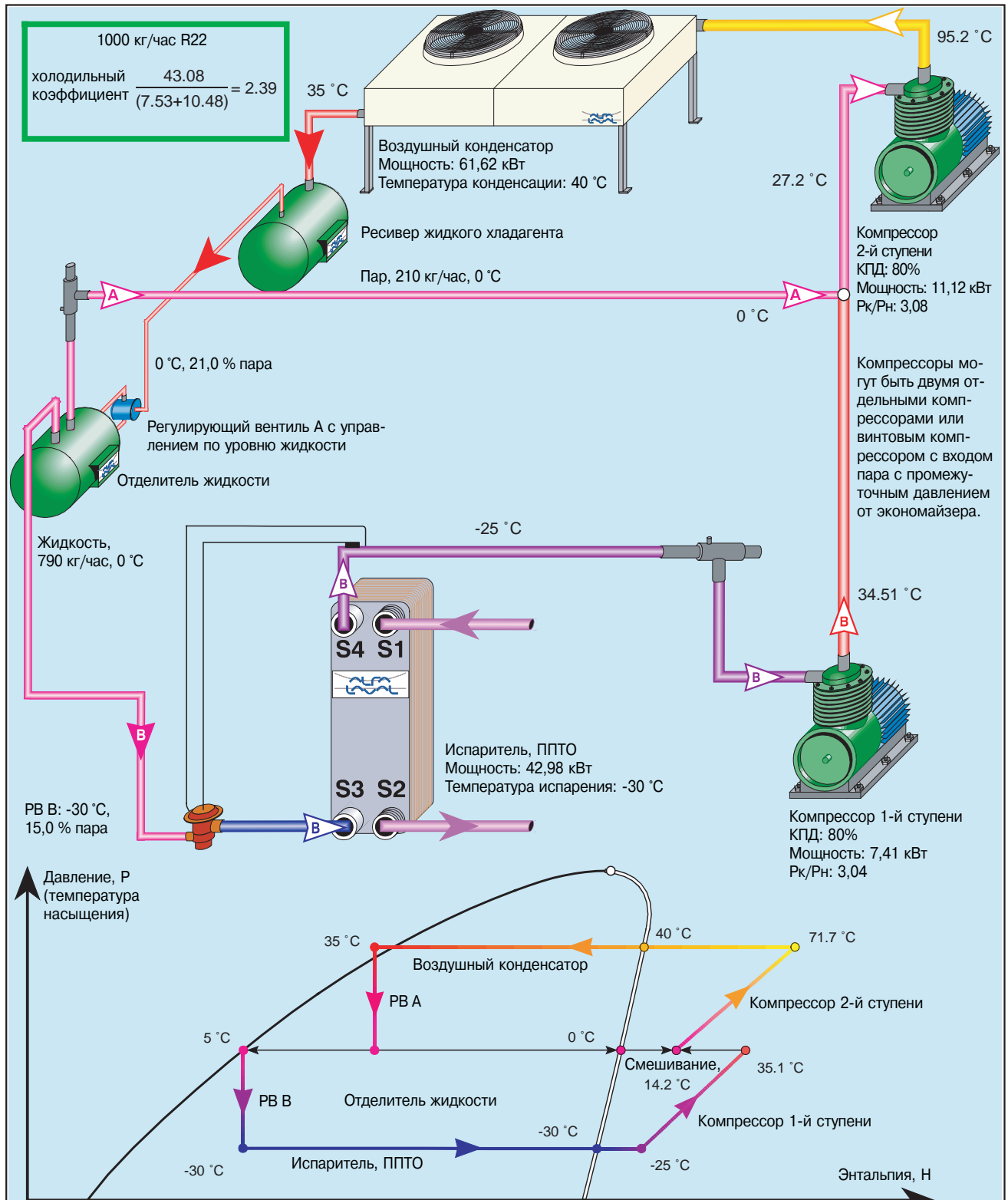
Рис. 03. Холодильный цикл с экономайзером мгновенного испарения
