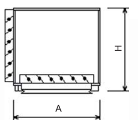
Смесительная камера
