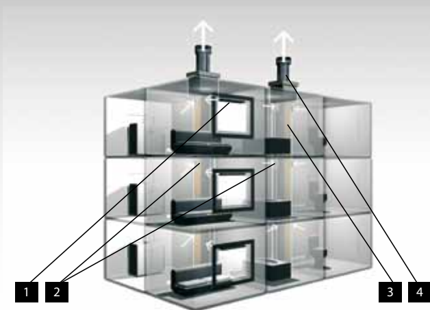
1. Приточные устройства 2. Вытяжные устройства 3. Вентиляционные каналы 4. Вентиляторы для поддержания работы естественной вентиляции
