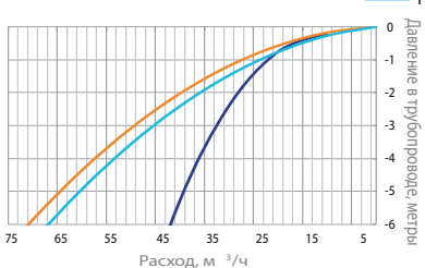
Впуск воздуха (свободный выход) 1/2", 3/4", 1"
