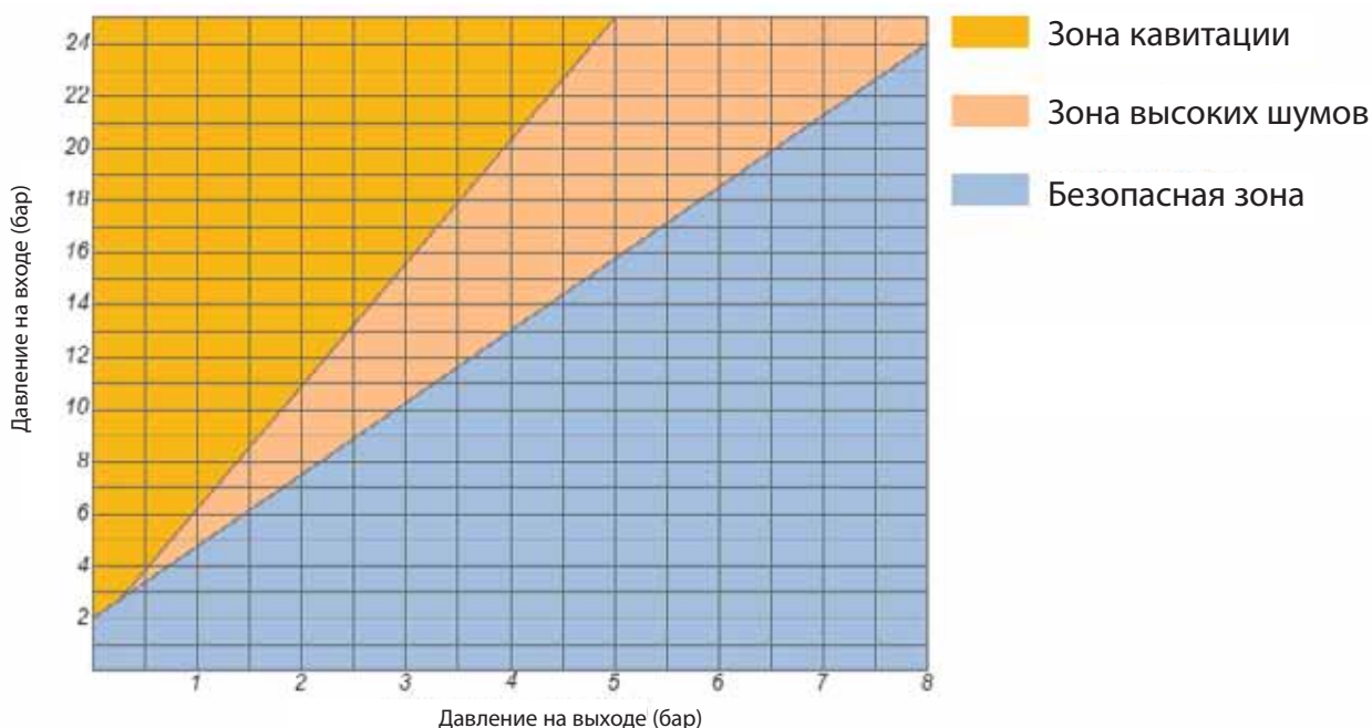
Диаграмма кавитации
