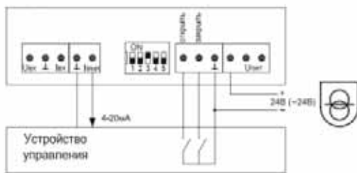
Схема подключения ЭИМ в режиме трехпозиционного управления (беспотенциальный контакт или открытый коллектор)
