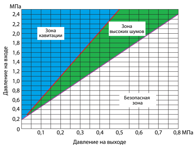
Данные по кавитации
