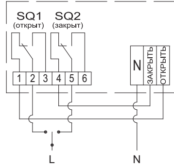
б) при работе с ограничением рабочего хода
