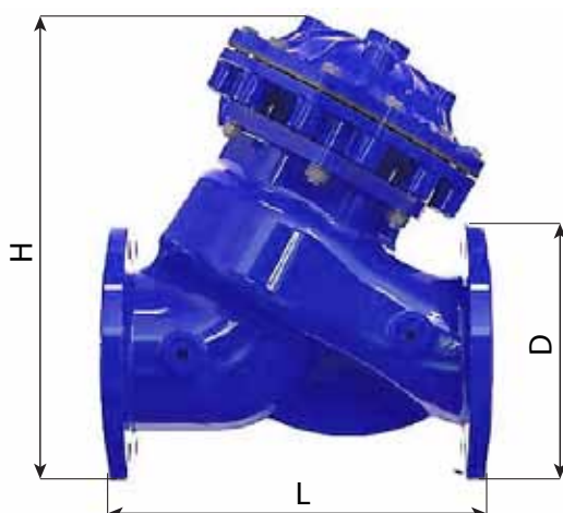
Габаритные размеры клапана: размеры (мм), масса (кг)
