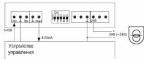
Схема подключения ЭИМ в режиме управления аналоговым сигналом 4-20 мА (0-10 В)
