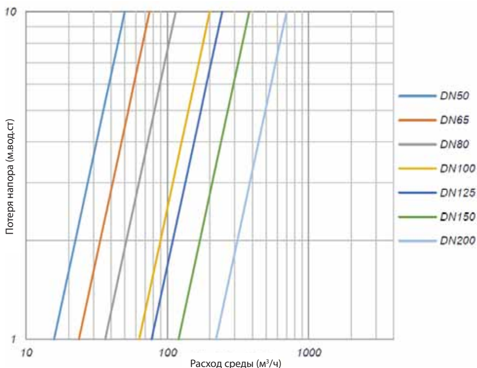
Диаграмма расхода
