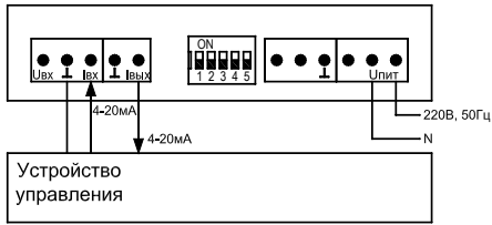
Схема подключения ЭИМ в режиме управления аналоговым сигналом 4-20 мА (0-10 В)
