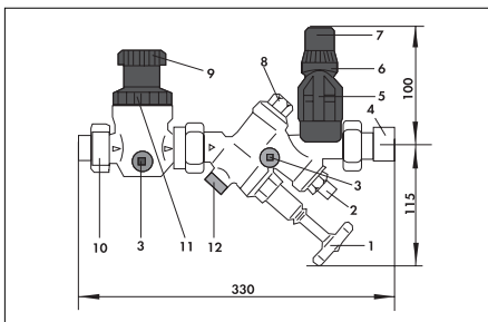
Рис.1 Элементы группы безопасности
