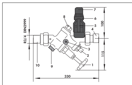
Рис.1 Элементы группы безопасности
