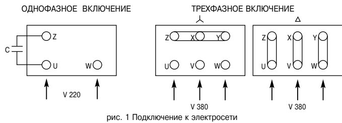
рис. 1 Подключение к электросети
