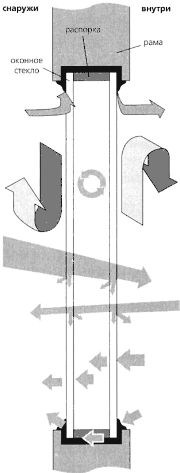
Рис. 5.16. Излучение и тепловые потоки в окне.
