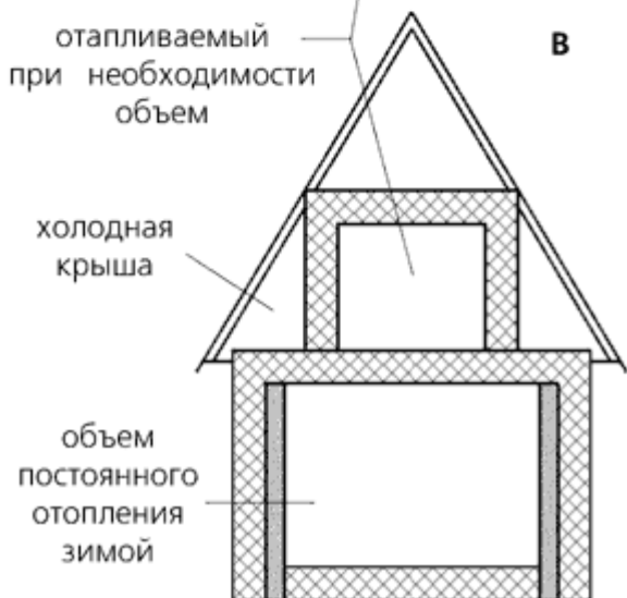
Рис. 5.3. Схемы утепления разных конструкций корпуса экодому.
