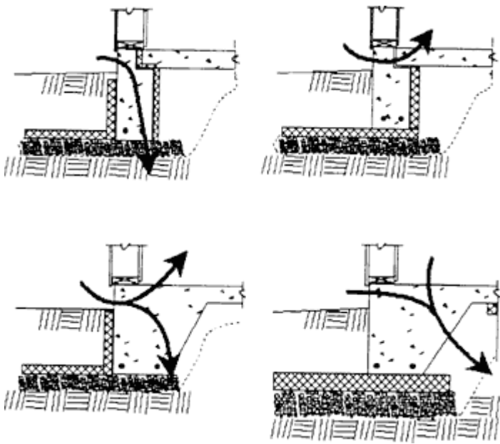
Рис. 5.10. Мостики холода.
