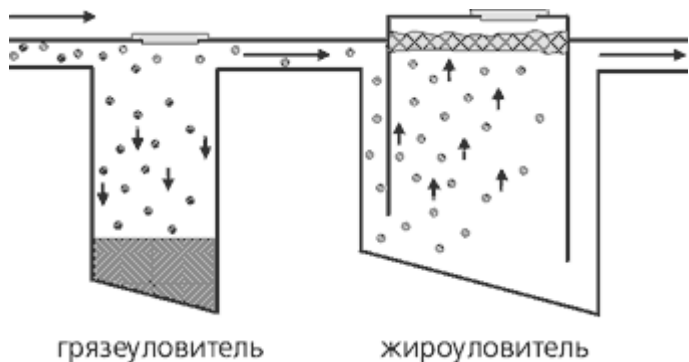
Рис. 12.5. Жируловитель.
