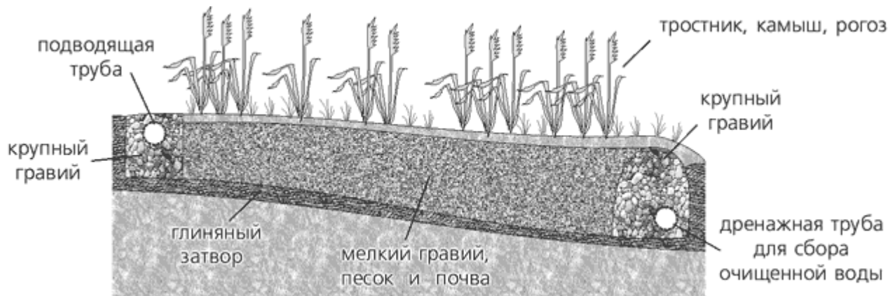
Рис. 12.11. Ботаническая площадка.
