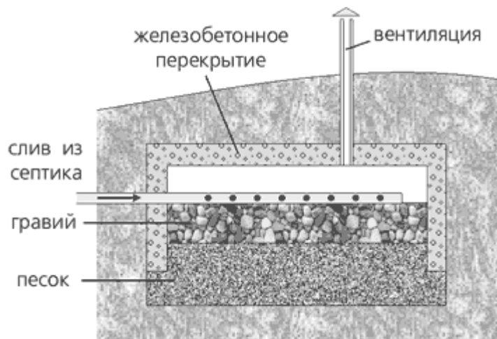
Рис. 12.9. Фильтрующая кассета.
