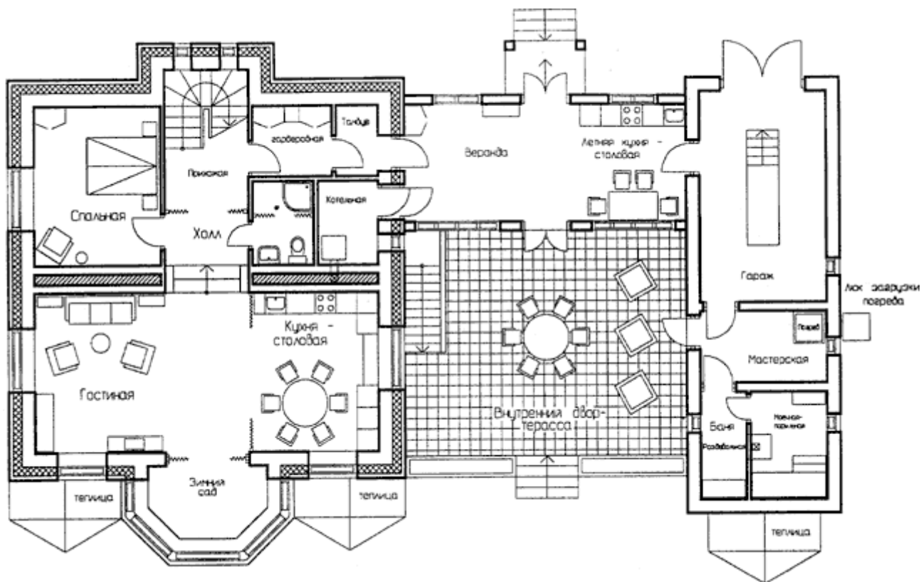
Рис. 4.3 Архитектура экоддома-подворья из разных строений. Эскиз. Планировка. (Проект А. Никитина)
