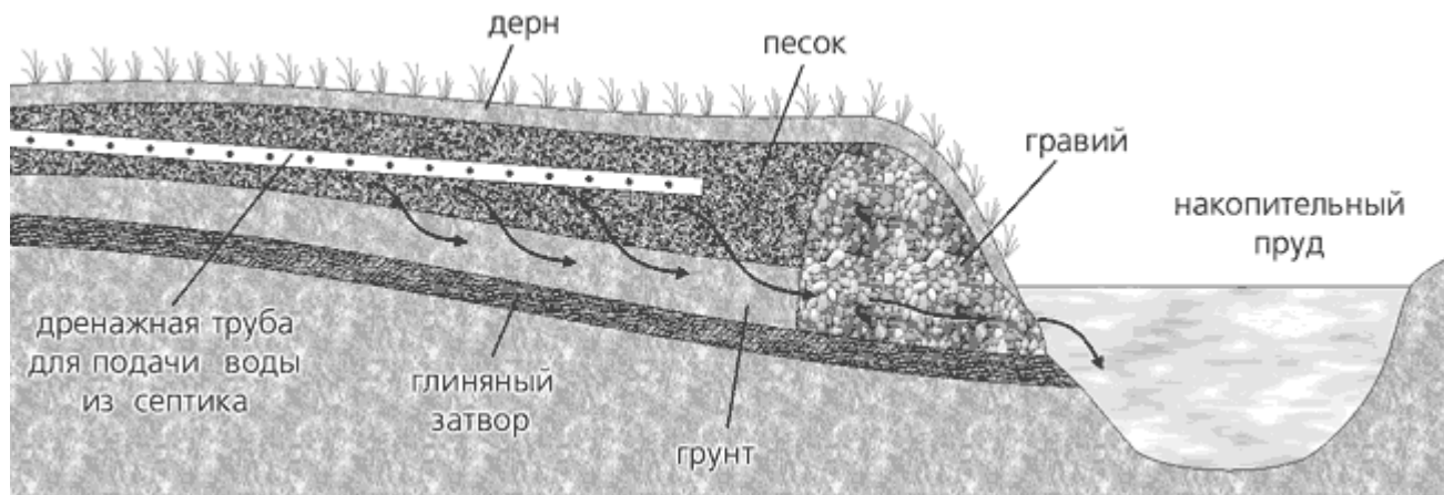
Рис. 12.10. Почвенно-песчаный фильтр.
