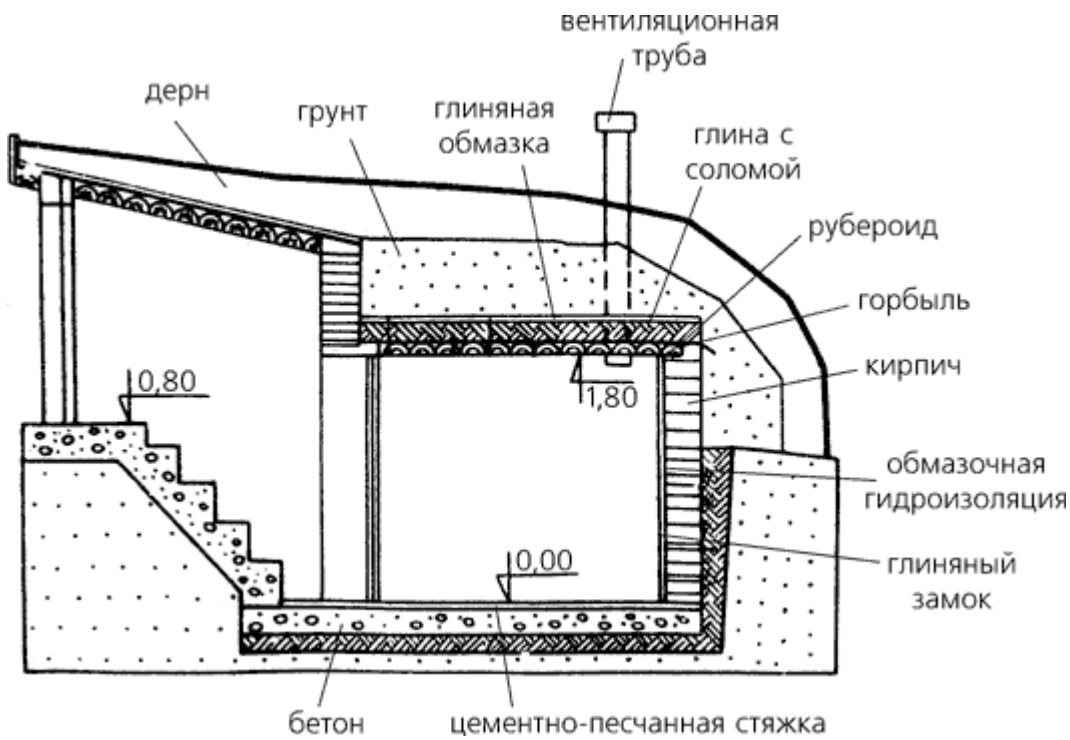
Рис. 7.2. Устройство погреба.
