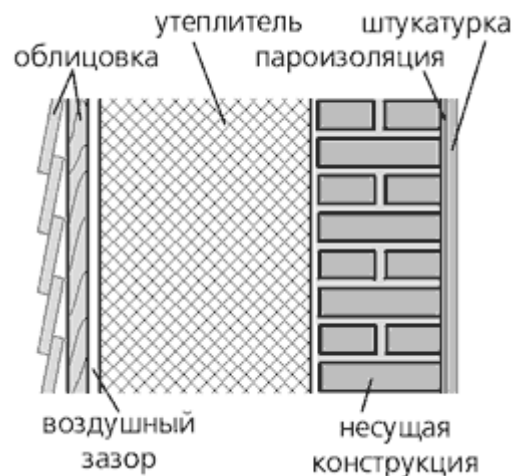
Рис. 5.12. Конструкция стены экодому.
