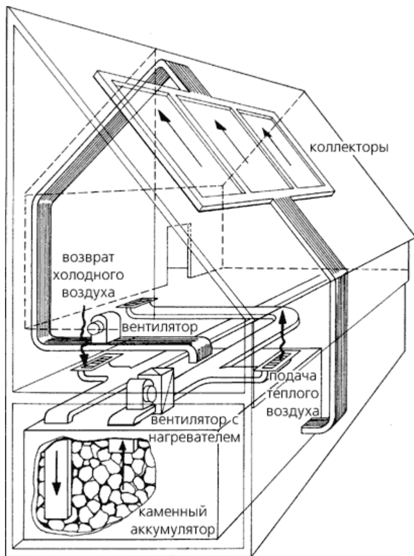
Рис. 6.1. Воздушная система солнечного обогрева с принудительной вентиляцией.
