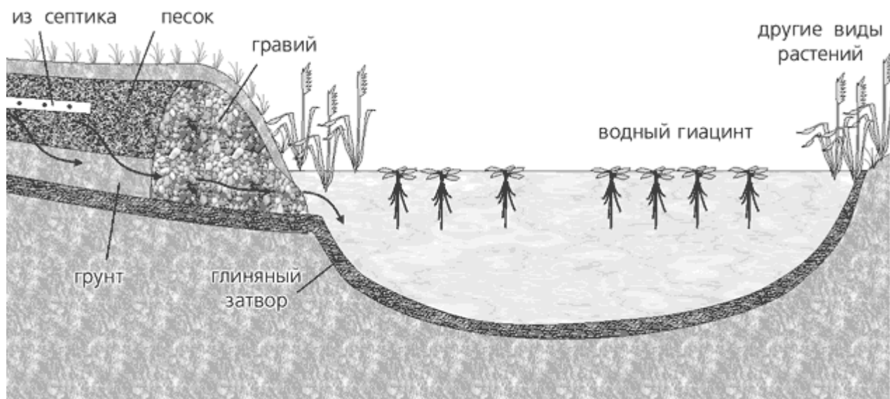
Рис. 12.12. Накопительный пруд.
