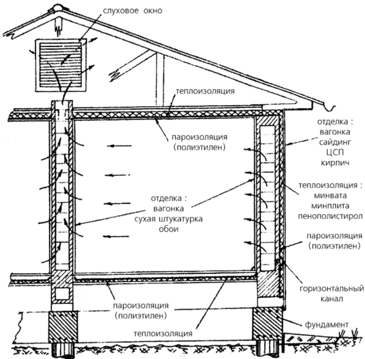
Рис. 8.2. Вытеснительная схема вентиляции.
