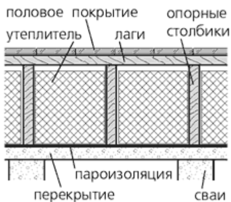
Рис. 5.11. Перекрытие первого этажа: а) по грунту б) над вентилируемым подпольем.
