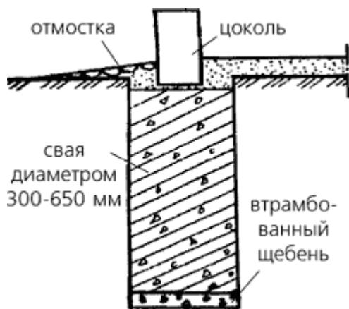
Рис. 5.5. Бутонабивной фундамент.
