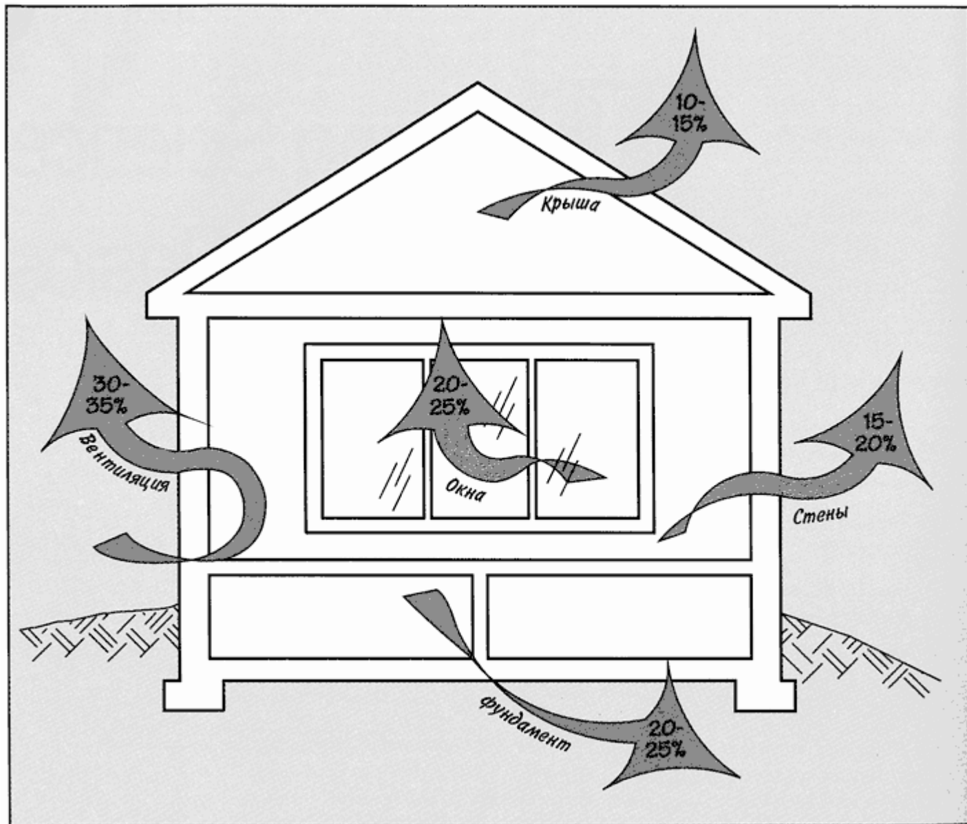
Рис. 5.1. Теплопотери через разные элементы ограждающей конструкции экодому.
