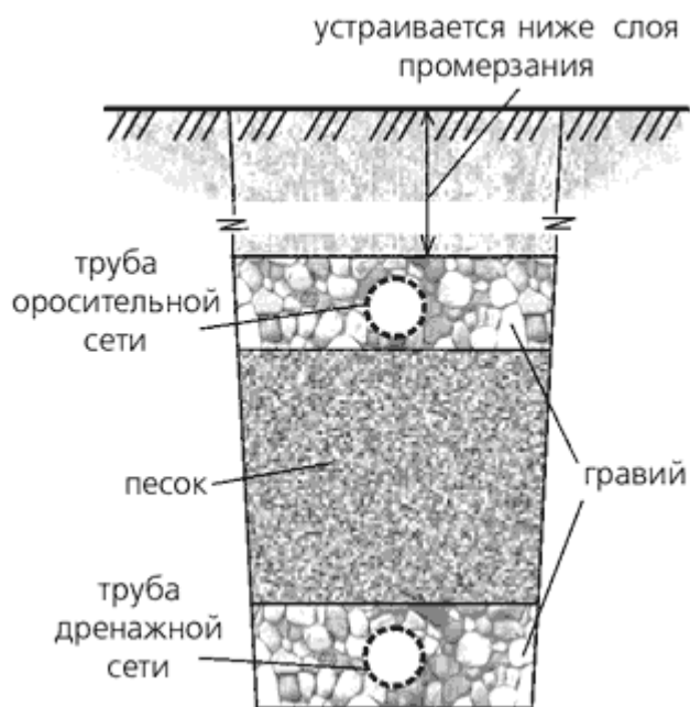
Рис. 12.8. Фильтрующая траншея.
