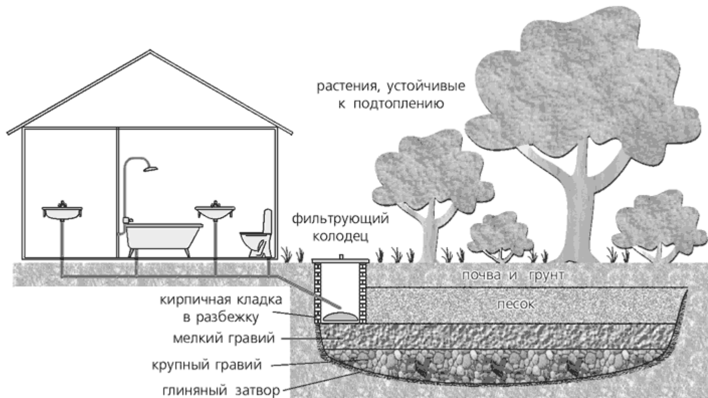
Рис. 12.1. Простейшая система накопительного типа с утилизацией смешанных стоков.
