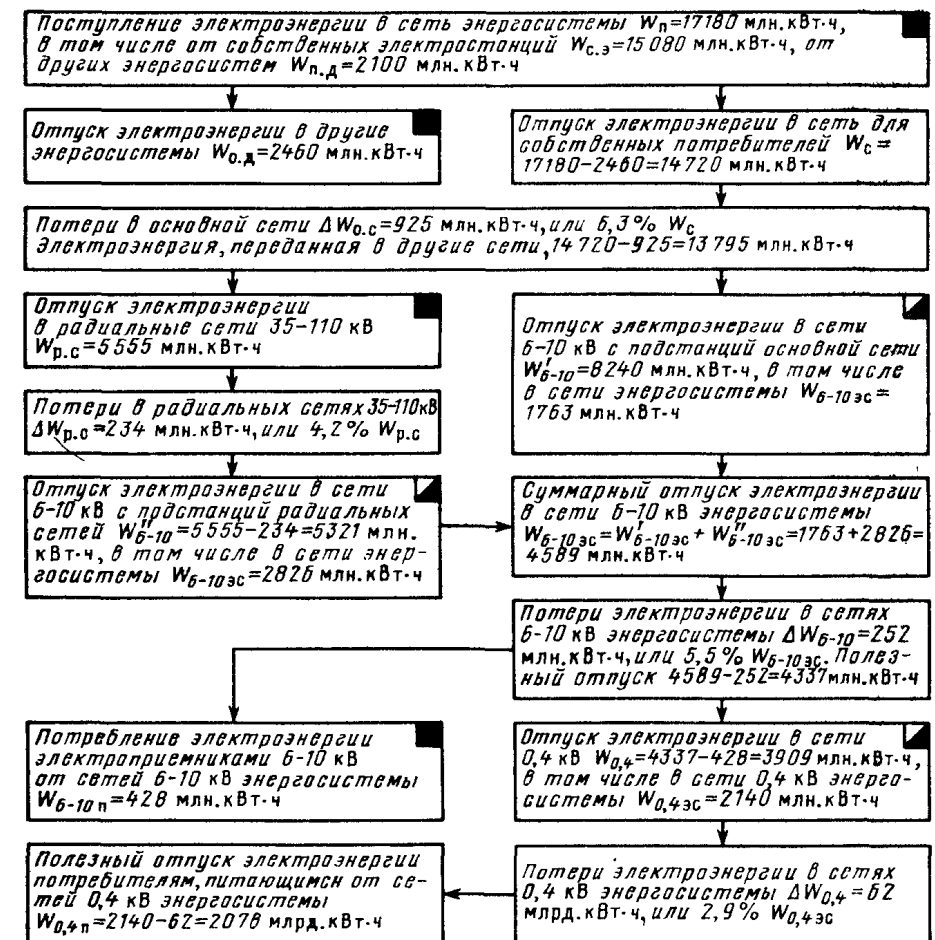
Рис. 2.1. Баланс электроэнергии по энергосистеме
