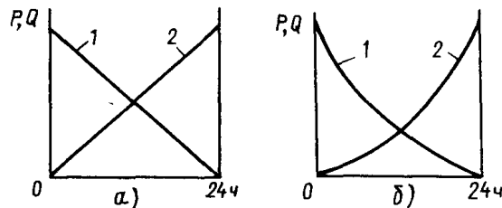
Рис. ПЗ.2. Идеализированные графики нагрузки узлов схемы рис. ПЗ.1
