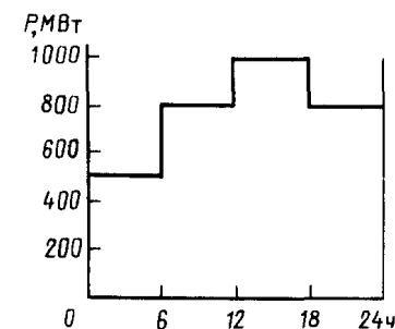
Рис. 3.5 Суточный график нагрузки энергосистемы
