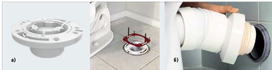
•• Фото 3. Фланец с прокладкой и болтами для установки унитаза с вертикальным выпуском на канализационную трубу в США (а). Манжета для подключения унитаза с горизонтальным выпуском к канализационной трубе снаружи унитаза в Европе (б)
