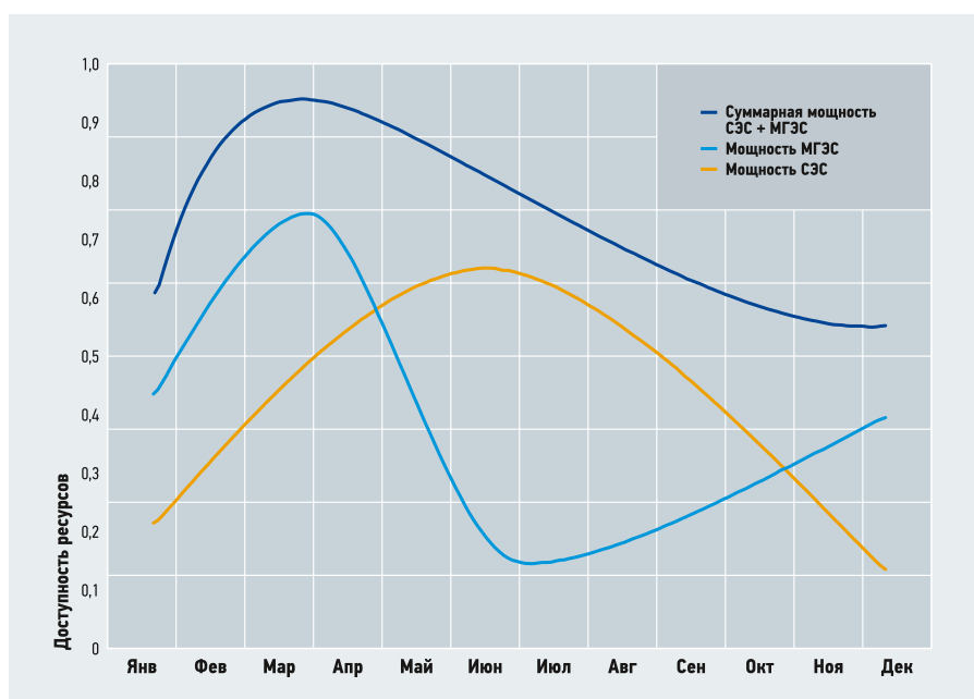
Рис. 6. Изменения суммарной мощности гибридной СЭС + МГЭС в гибридной энергосистеме на годовом отрезке времени [9]
