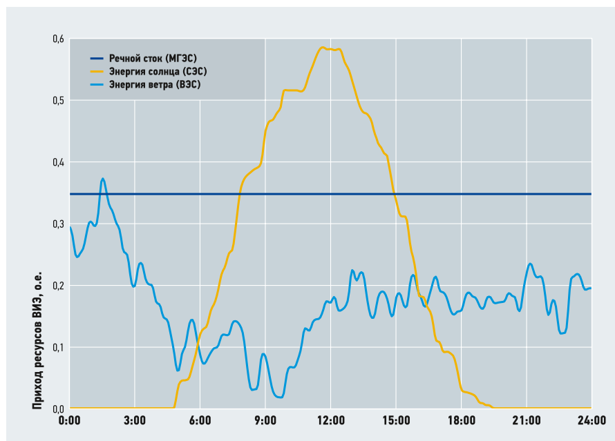
Рис. 4. Характер изменения прихода ресурсов ВИЭ в течение суток в условном районе [2]
