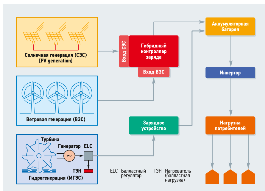
Рис. 9. Гибридная система возобновляемой энергетики [20]
