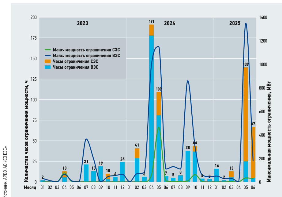
Рис. 5. Изменения максимальной мощности и количества часов ограничения мощности СЭС и ВЭС в энергосистеме [1]
