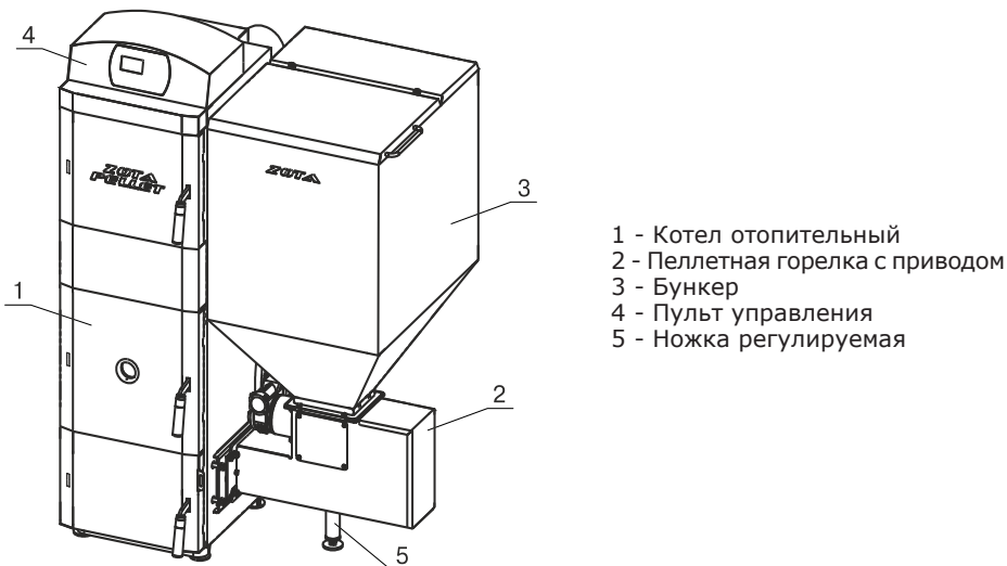
Рис.1. Котел пеллетный в сборе.
