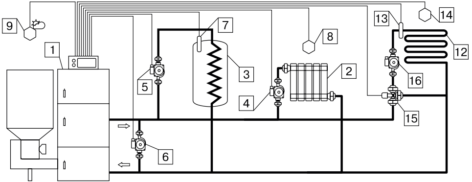
Рис.9. Упрощенная схема подключения котла с уломрециркуляции.
