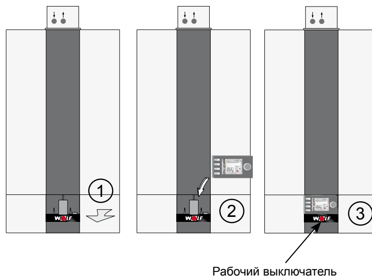
Рис. 4.1 Установка модуля управления VM-2 в СGB-2
