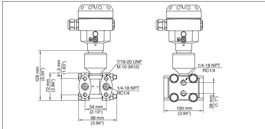
Рис. 63: DPT10, присоединение 1/4-18 NPT или RC 1/4, с выпуском воздуха сбоку
