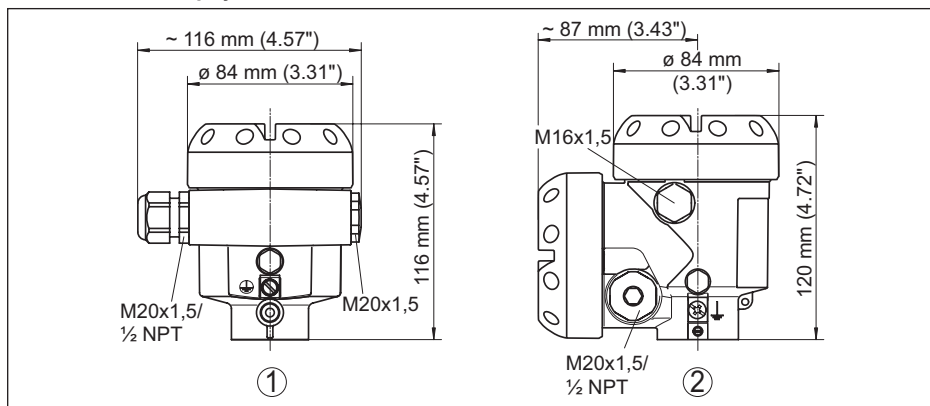
Рис. 59: Корпуса в исполнении IP 66/IP 68 (0,2 bar) - с установленным модулем индикации и настройки корпус выше на 9 мм/0.35 in
