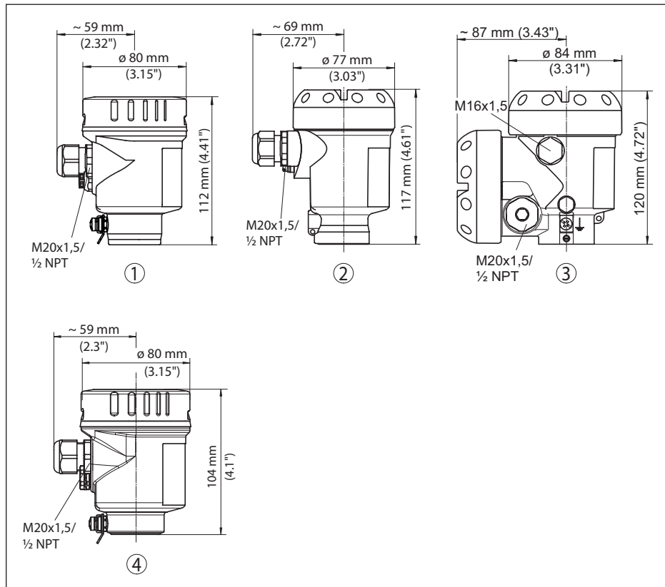
Рис. 61: Корпуса в исполнении IP 66/IP 68 (0,2 bar) - с установленным модулем индикации и настройки корпус выше на 9 mm/0.35 in
