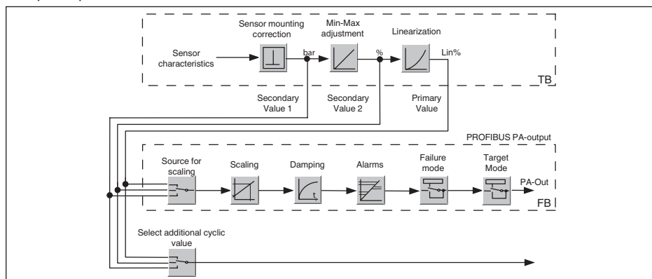
Рис. 51: DPT10: Блок-схема со значением AI (PA-OUT) и дополнительным циклическим значением (Additional Cyclic Value)
