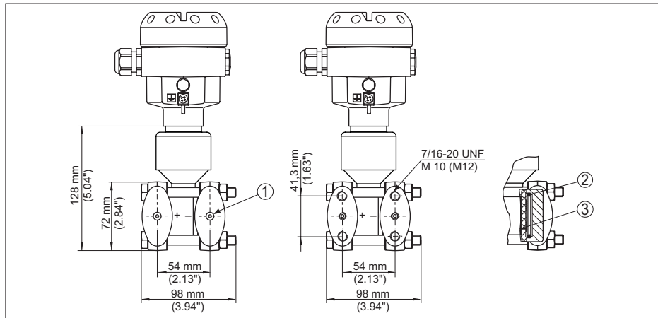
Рис. 64: Слева: Присоединение DPT10 подготовлено для монтажа изолирующей диафрагмы. Справа: Положение медного уплотнительного кольца
