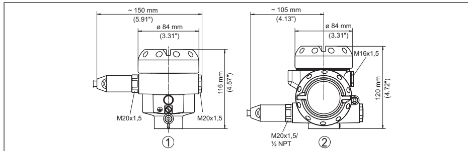
Рис. 60: Корпуса в исполнении IP 66/IP 68 (1 bar) - с установленным модулем индикации и настройки корпус выше на 9 мм/0.35 in
