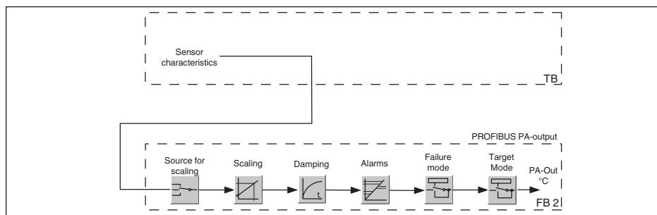
Рис. 52: DPT10: Блок-схема со значением температуры
