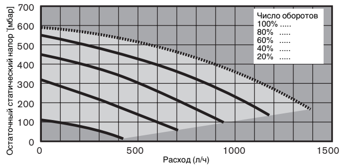
Диаграмма остаточного статического напора системы WTC 15-A Котракт с 3-ступенчатым насосом
