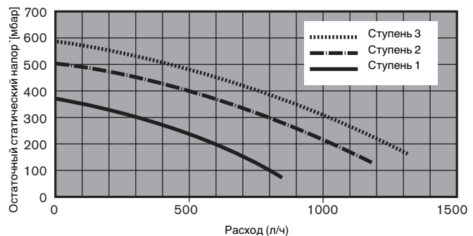
Диаграмма остаточного статического напора системы WTC 25-A Котракт с 3-ступенчатым насосом
