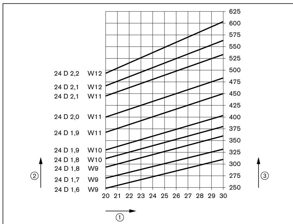
Диаграмма подбора форсунок
