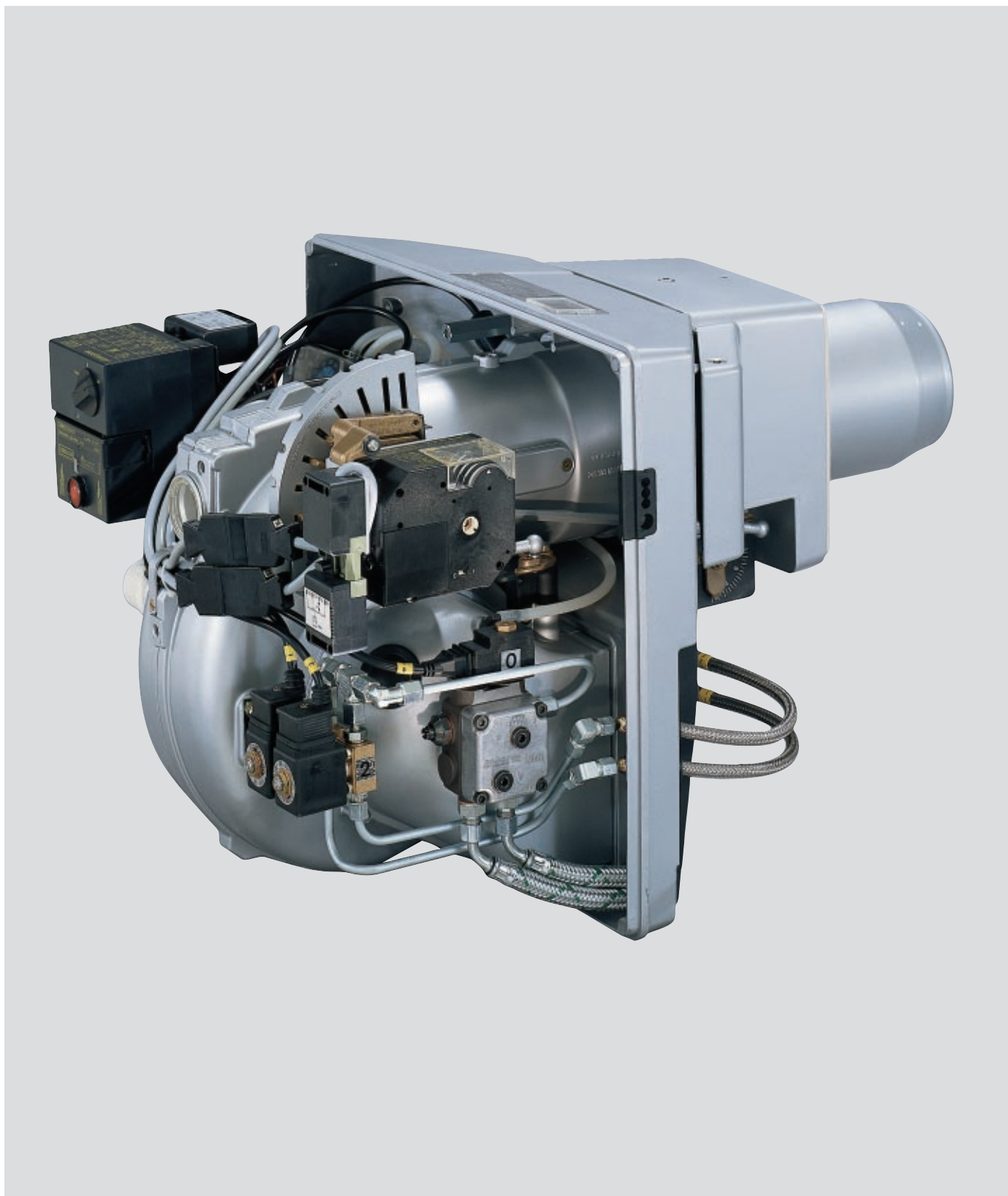
Комбинированная горелка WGL30 (без кожуха)
