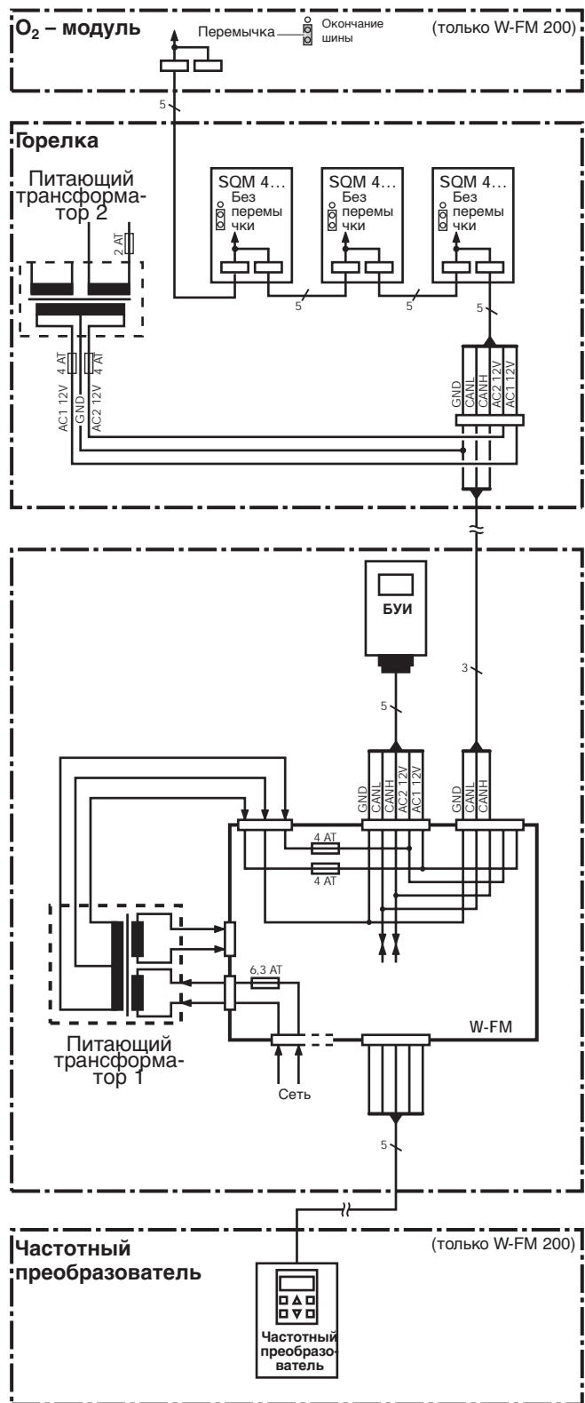
Пример монтажа: W-FM в шкафу управления
