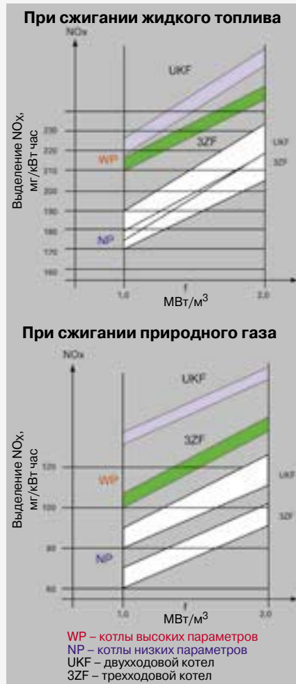
Образование \text{NO}_x в зависимости от теплового напряжения камеры сгорания и конструкции котла для жидкого топлива и природного газа
