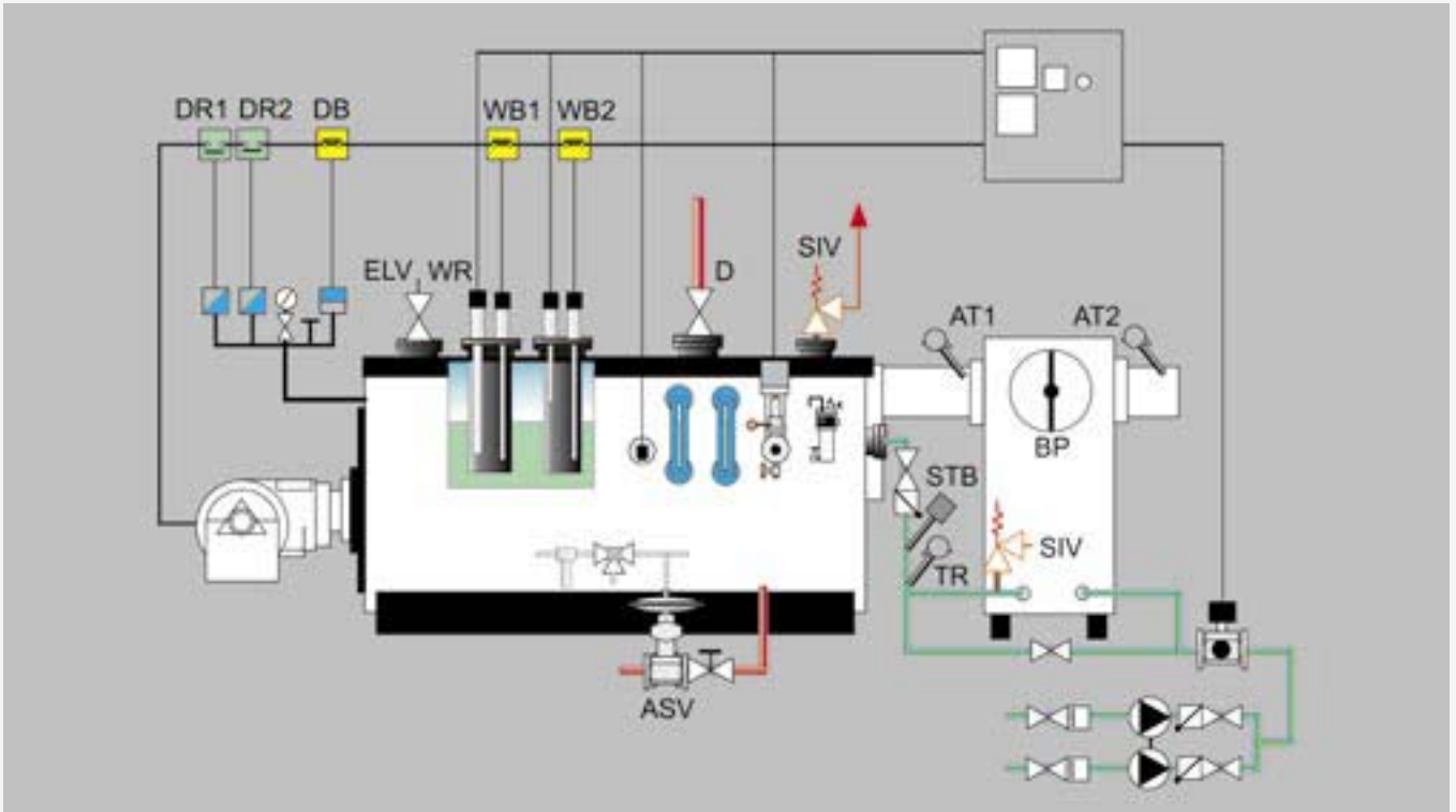
Основное оборудование парового котла высокого давления серии Vitomax 200 HS с экономайзером
