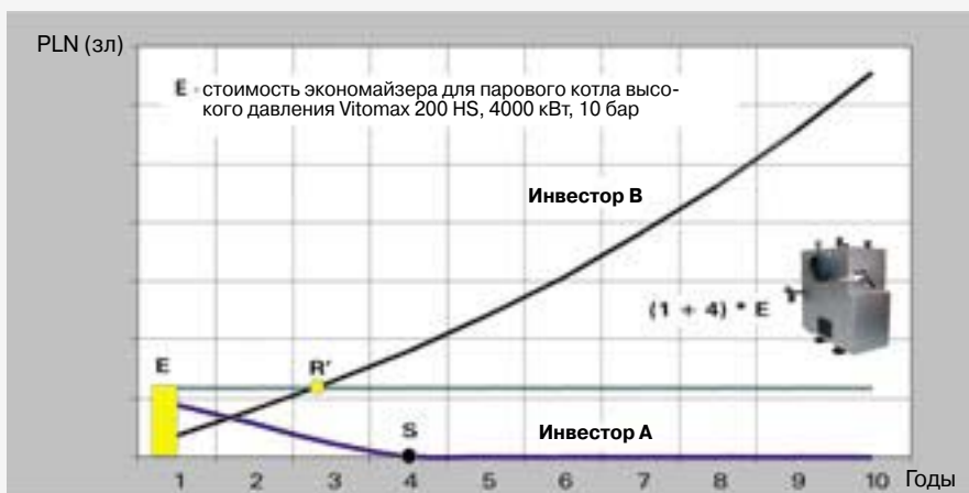
Варианты капиталовложений E Инвестор А — отказ от экономайзера. Инвестор В — установка экономайзера
