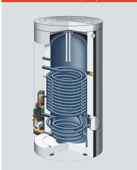
Рис. D.1.4–2 Емкостный водонагреватель
