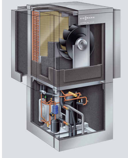
Рис. А.3.3–2 Воздушно-водяной насос
