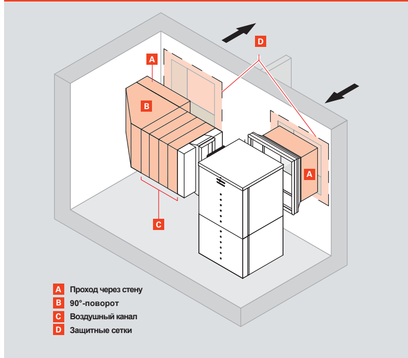
Рис. С.3.4–1 Забор воздуха для внутренней установки
