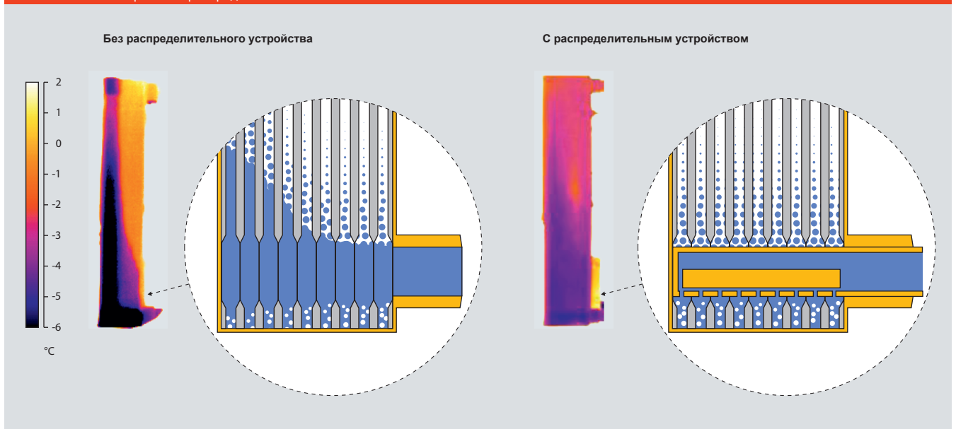
Термографические снимки наглядно показывают распределение тепла в теплообменном аппарате без распределительного устройства (слева), когда хладагент неравномерно покрывает поверхность теплообмена и с распределительным устройством (справа).
