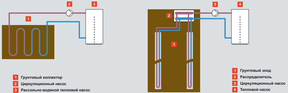
Рис. С.1.1-1 Грунтовый коллектор и грунтовый зонд
