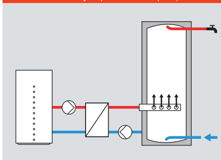
Рис. D.2.1-15 Функциональный принцип
