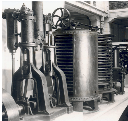
Рис. А.1–3 Холодильная машина Линда 1877 года
