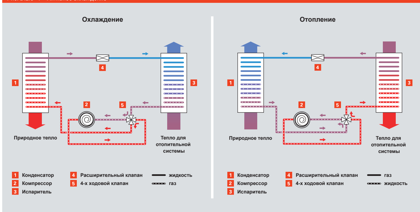
Рис. D.2.3-4 Активное охлаждение
