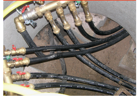
Abb. A.4.1–8 Soleverteiler bei Erdsonden
