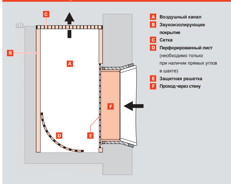
Рис. С.3.4–2 Поток воздуха в канале
