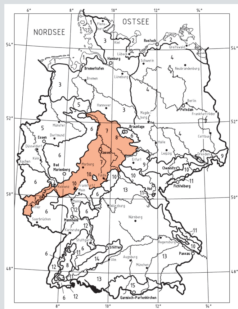
Рис. С.1.1–5 Климатическая карта по DIN 4710
