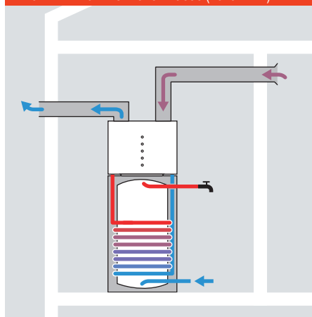
Рис. D.2.1–10 Тепловой насос (поточный)
