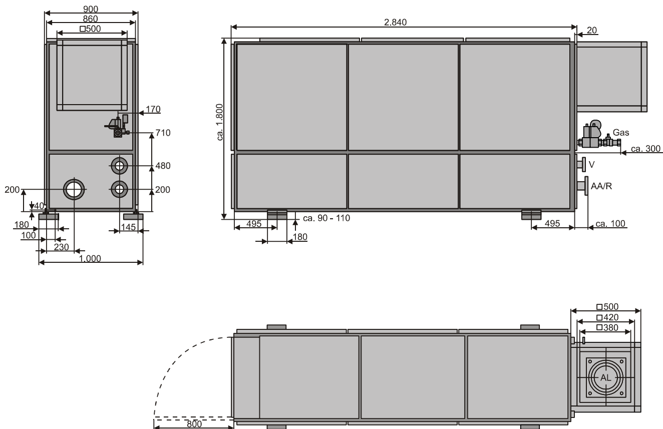
Рис. 1 Габаритные и присоединительные размеры VITOBLOC 200 EM-70/115 (размеры в мм); Установленный короб вентилятора на задней панели можно демонтировать для транспортировки модуля.
