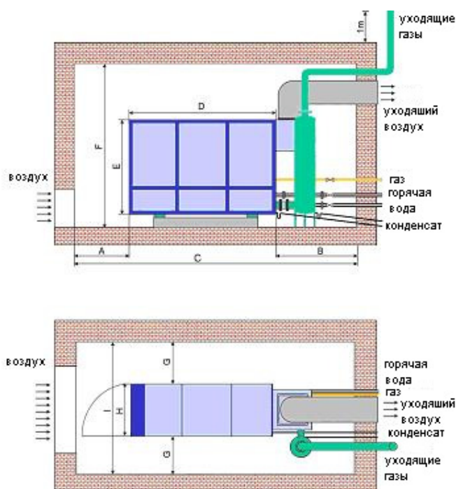
Рис.6 Необходимые расстояния в помещении (размеры в мм)
