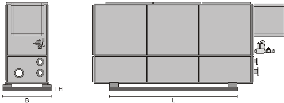
Размеры цоколя модуля VITOBLOC 200 EM-70/115
