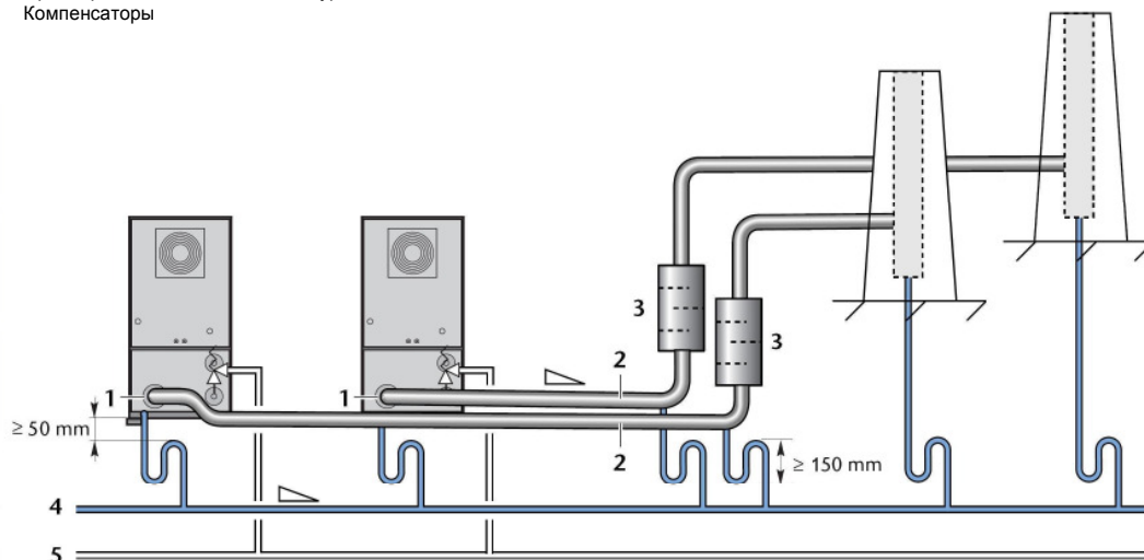
Рис. 9 Схема внешней системы выхлопных газов для двух модулей с отводом конденсата и дренажом предохранительных клапанов (размеры в мм)
