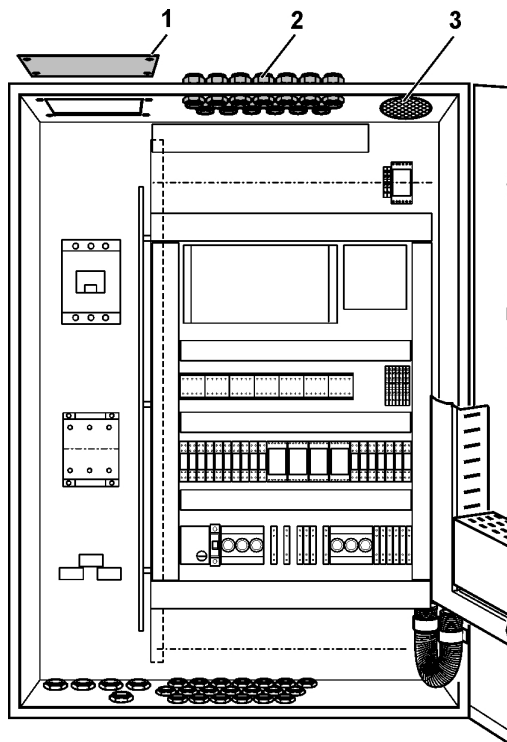
Рис. 12 Подвод кабеля к электрощиту модуля
