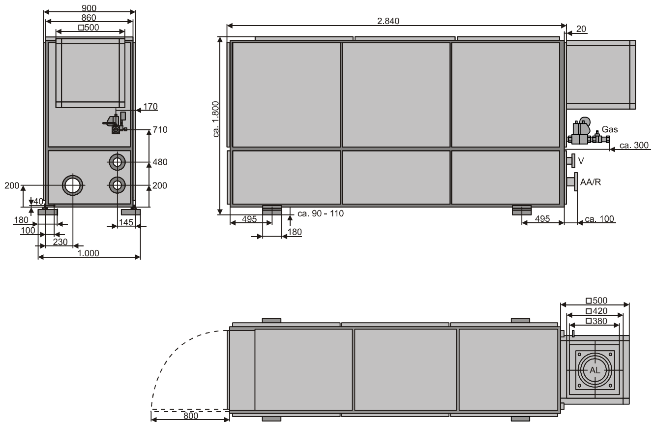
Рис. 1 Габаритные и присоединительные размеры VITOBLOC 200 EM-50/81 (размеры в мм); Установленный короб вентилятора на задней панели можно демонтировать для транспортировки модуля.
