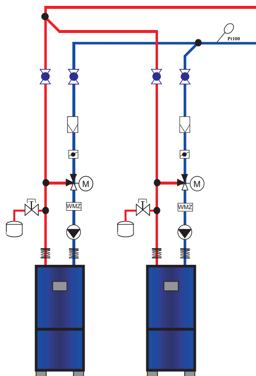
Рис. 10 Схема гидравлических подключений
