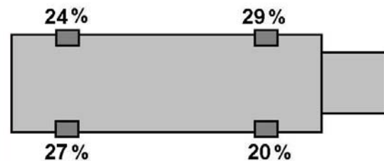
Рис. 3 Распределение нагрузки на опоры
