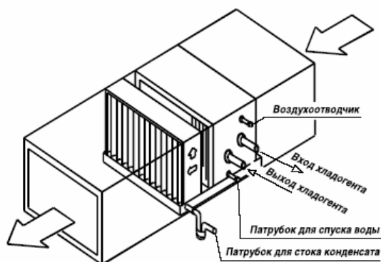
Подвод теплоносителя с патрубками нагревателя с левой стороны
