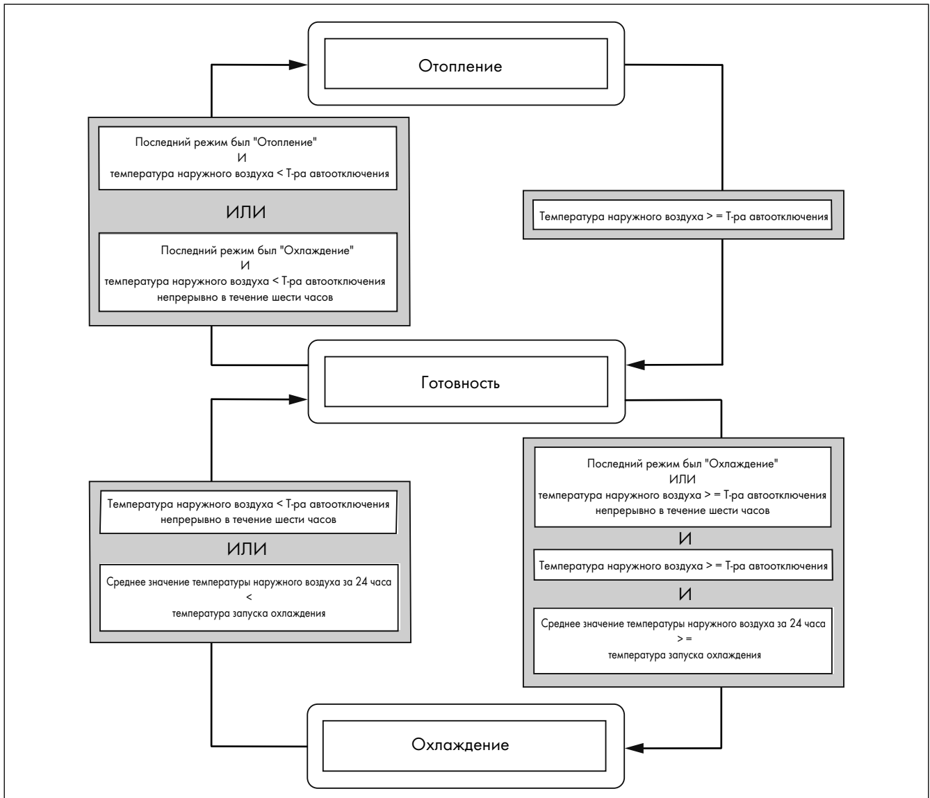
3.4 Схема перехода
