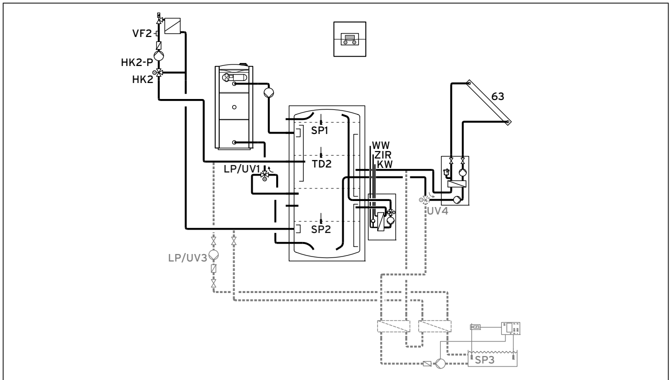
5.37 Гидравлическая схема 9.2
