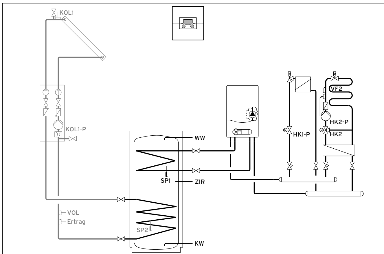
5.15 Гидравлическая схема 3.3
