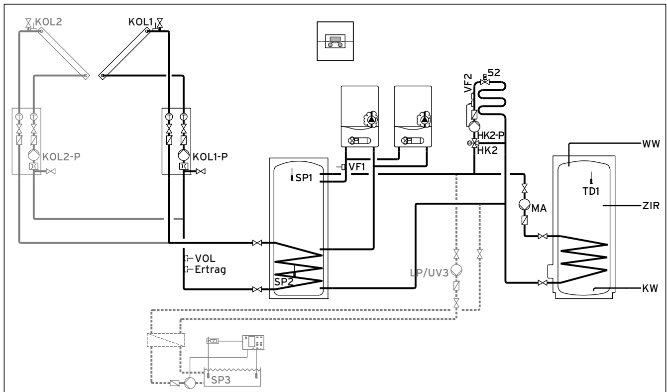
5.25 Гидравлическая схема 5.2
