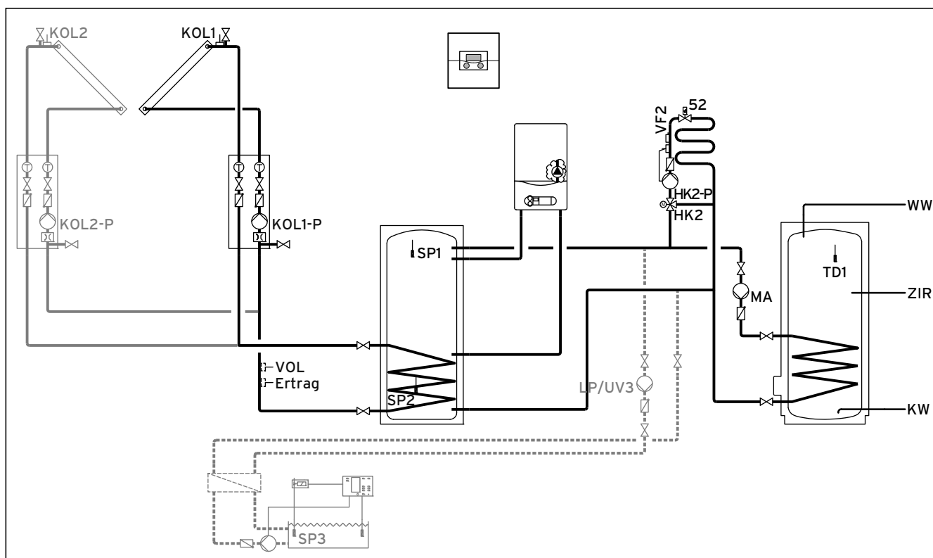
5.23 Гидравлическая схема 5.1
