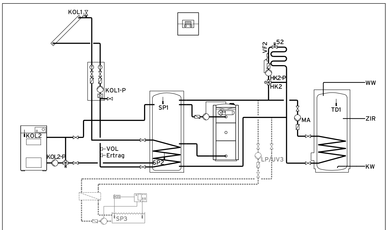
5.33 Гидравлическая схема 8
