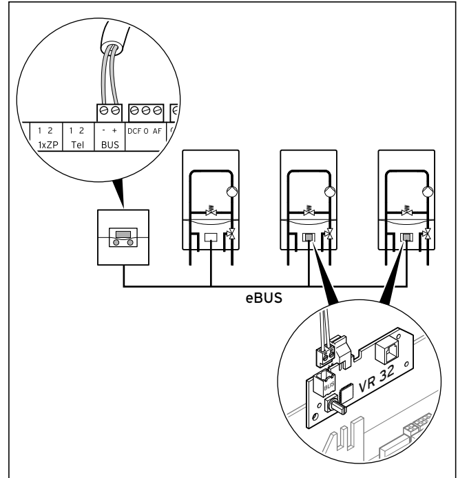
5.46 Подключение каскада из более чем 2 отопительных аппаратов
