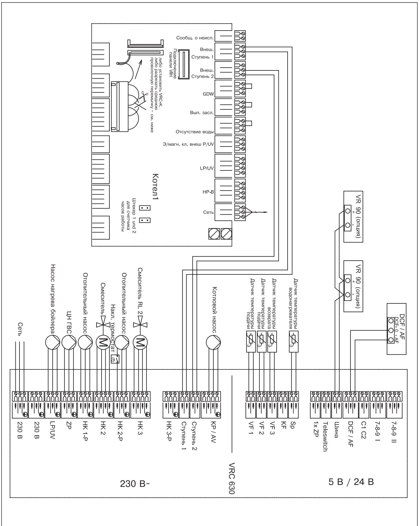
Рис. 4.13: Монтаж присоединительных проводов к VRC 630: котёл GP 210 с регулированием температуры обратной линии, 1 ВИН, 2 контура отопления
