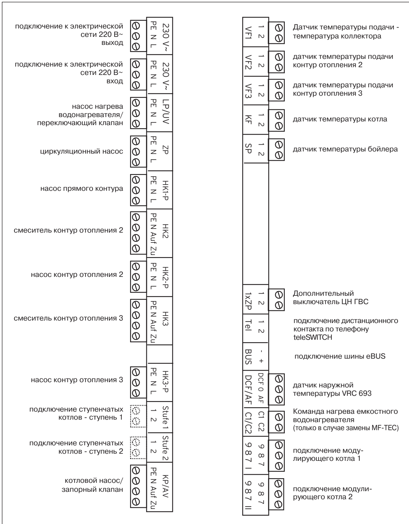
Рис. 4.3: Разводка контактов
