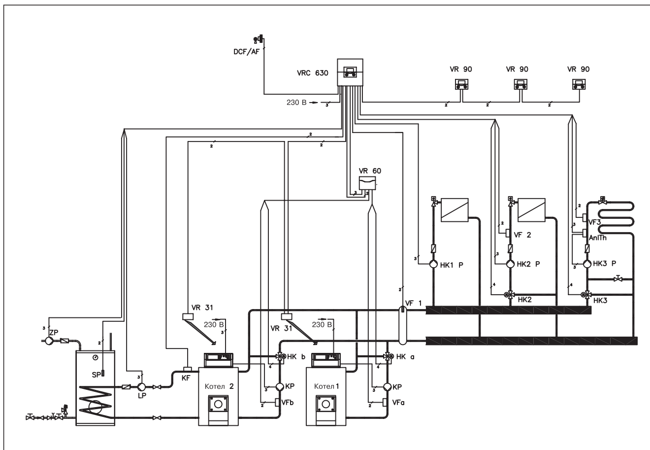
Рис. 4.14: VRC 630 с модулем VR 60: каскад из 2 GP 210 с отдельным включением водонагревателя ViH, 3 контура отопления
