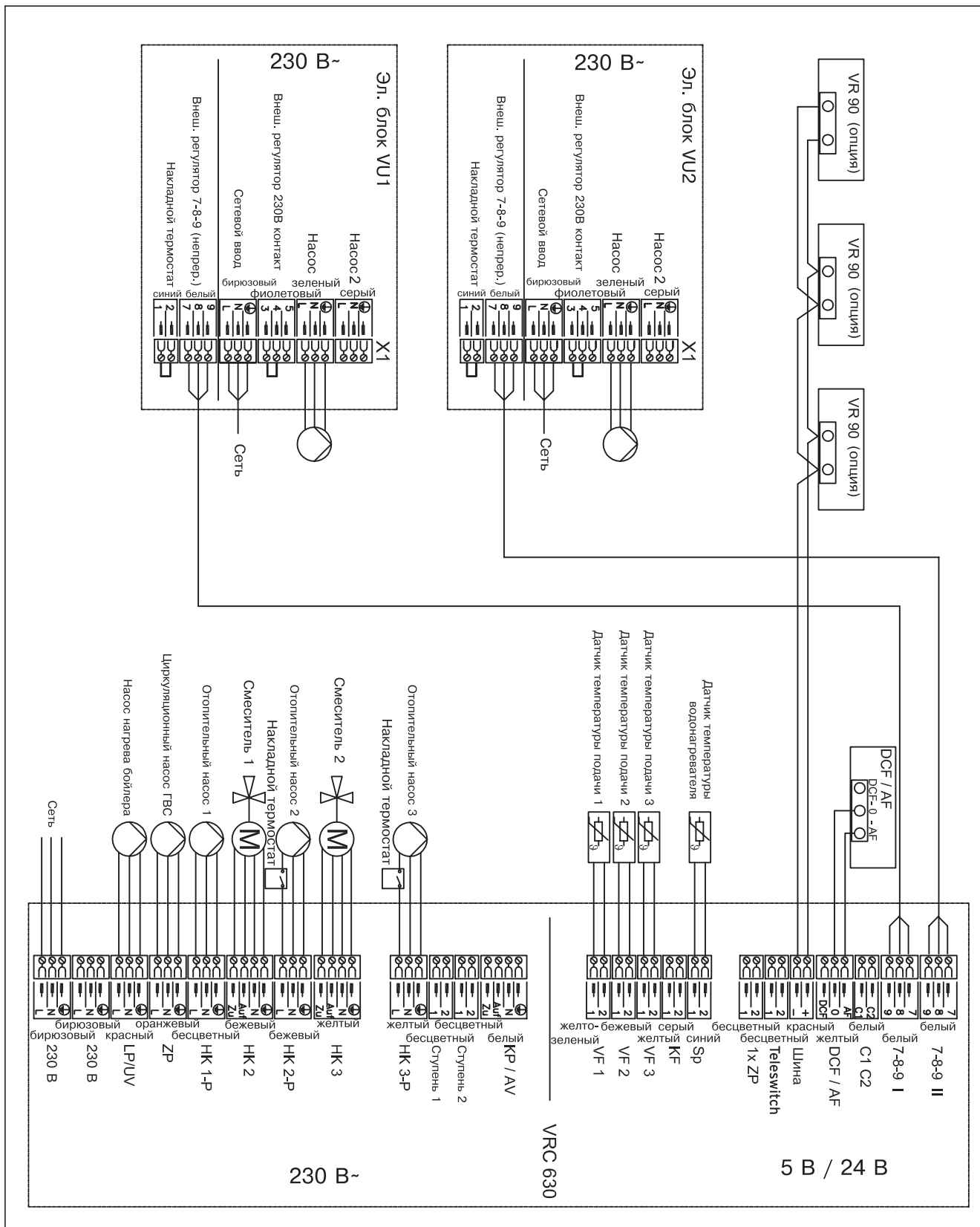
Рис. 4.7: Монтаж присоединительных проводов к VRC 630: 2 VU, 3 контура отопления, 1 VIH
