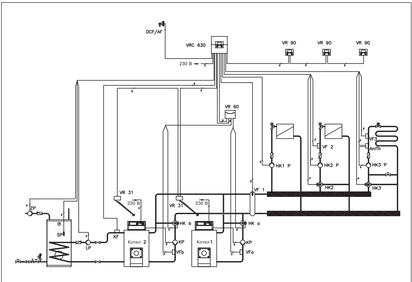
Рис. 4.14: VRC 630 с модулем VR 60: каскад из 2 GP 210 с отдельным включением водонагревателя VIH, 3 контура отопления
