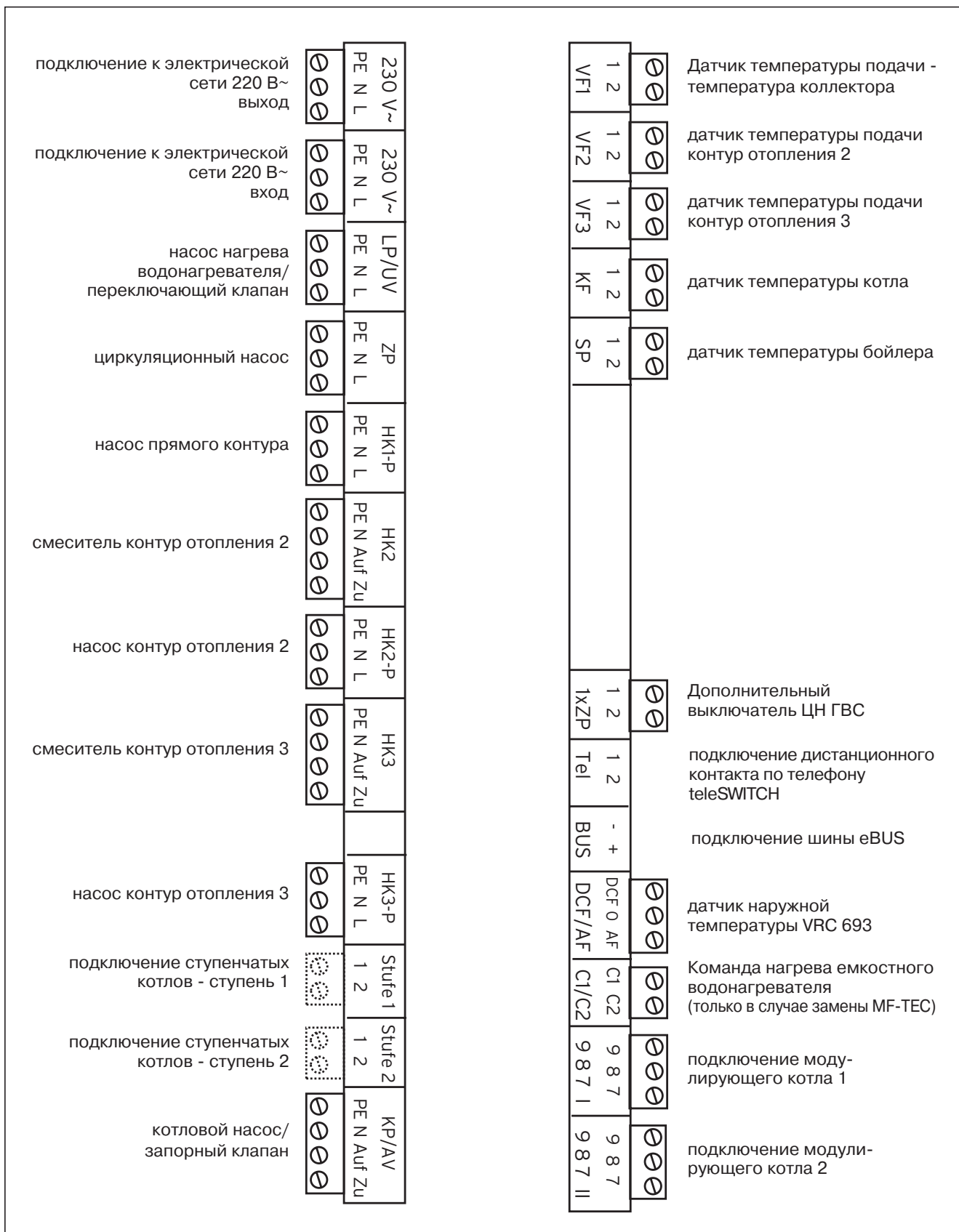
Рис. 4.3: Разводка контактов
