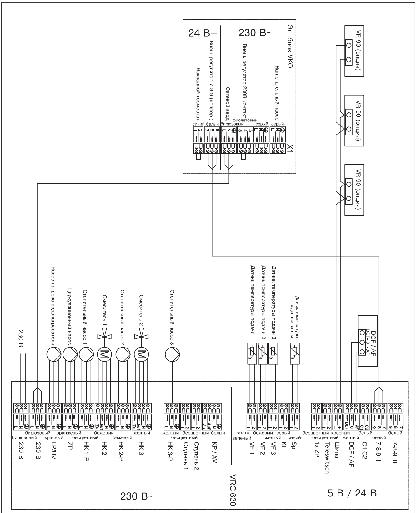
Рис. 4.11: Монтаж присоединительных проводов к VRC 630 и напольному котлу VKO
