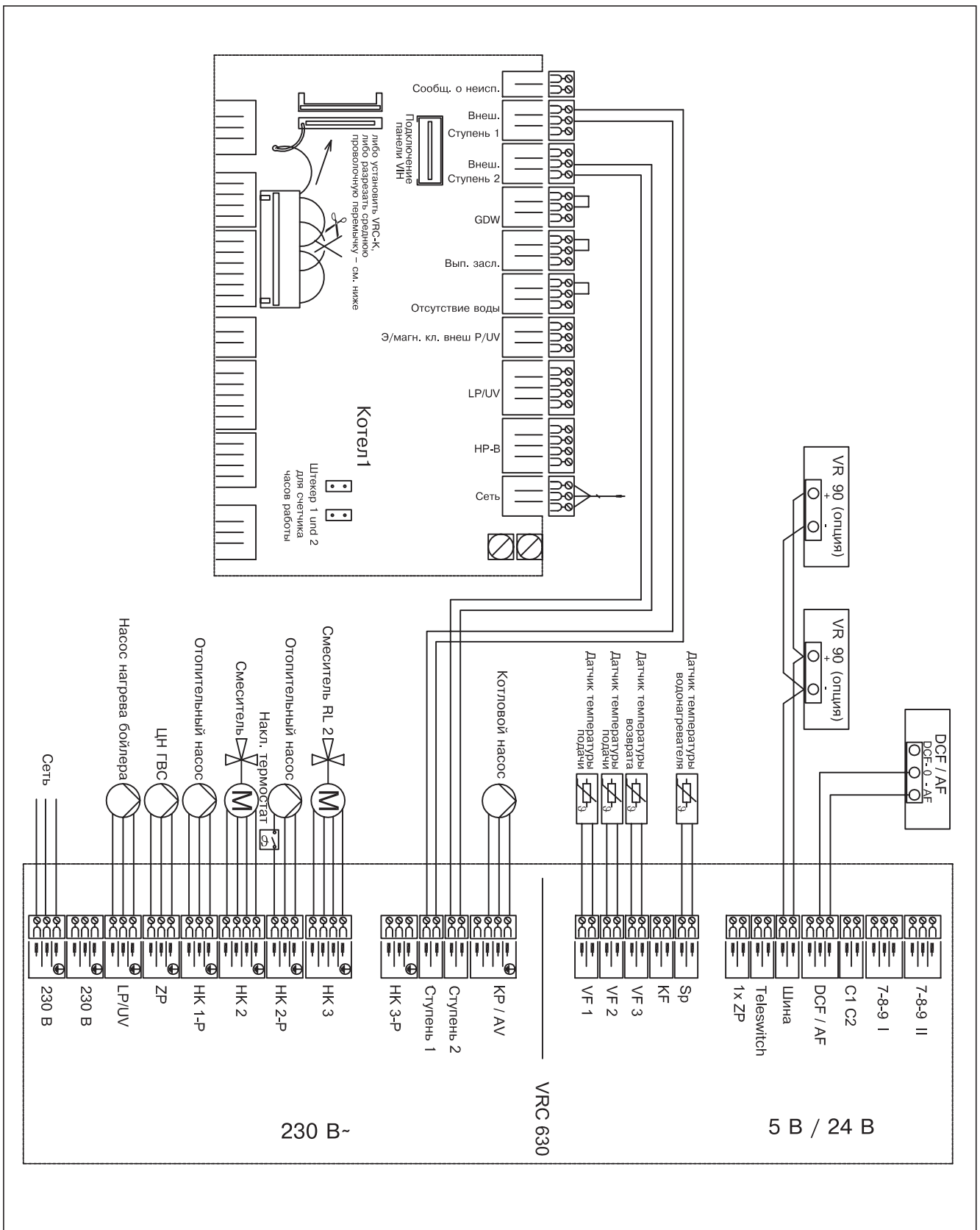
Рис. 4.13: Монтаж присоединительных проводов к VRC 630: котёл GP 210 с регулированием температуры обратной линии, 1 VIH, 2 контура отопления
