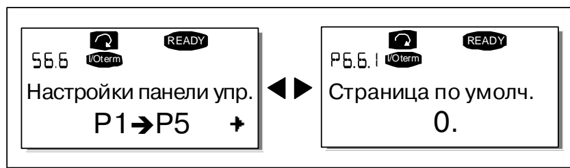
Рисунок 7-18. Подменю Настройки панели управления
