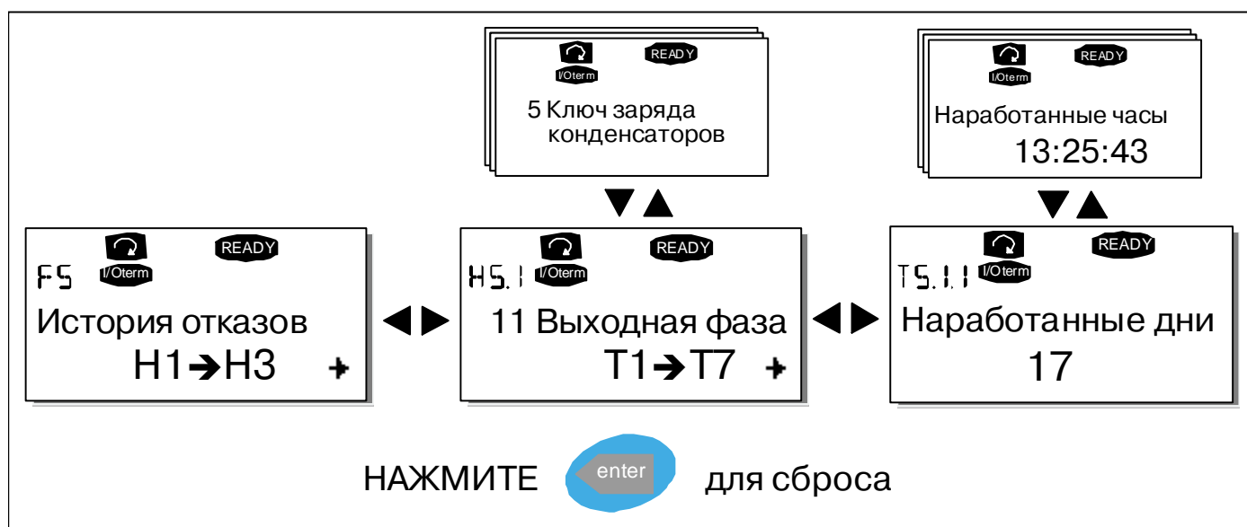
Рисунок 7-8. Меню Истории отказов
