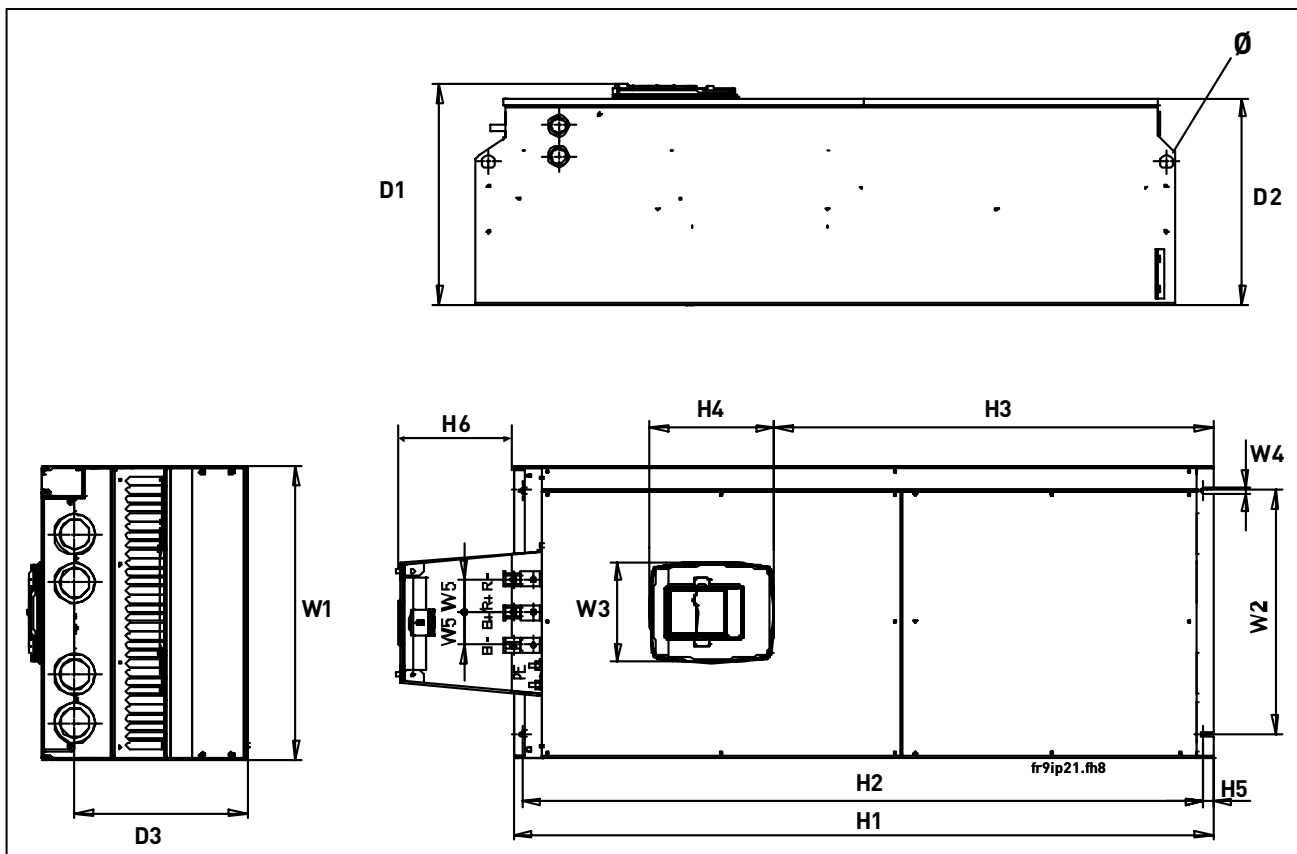
Рисунок 5-7. Габариты преобразователей частоты Vacon NX, типоразмер FR9
