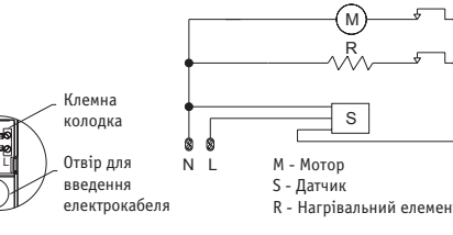
Мал. 7 Електросхема
