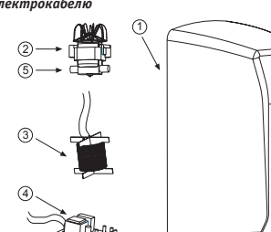
Мал. 9 Огляд компонентів 1 - Кришка 2 - Мотор з вентилятором 3 - Нагрівальна спіраль 4 - Електронна плата 5 - Щітки
