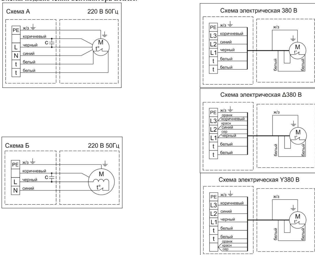
Рисунок 2. Схемы подключения вентилятора ВКПН:
