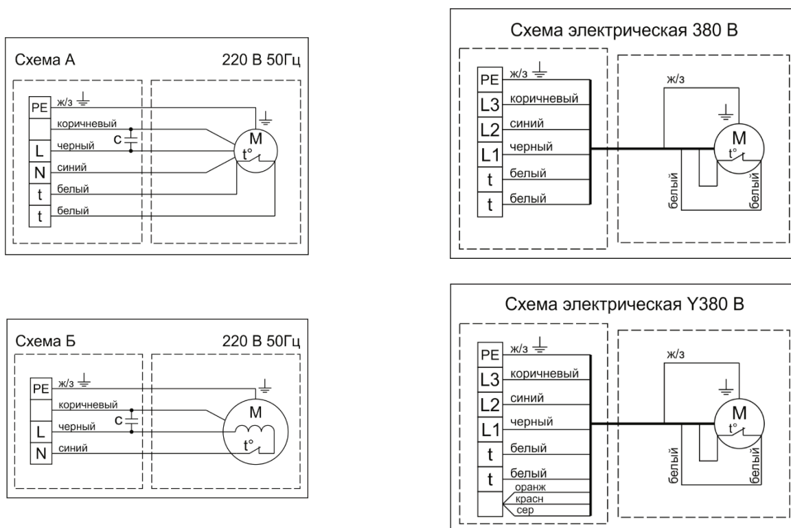
Рисунок 2. Схемы подключения вентилятора ВКП:
