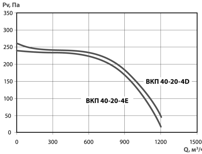
Рисунок 3. Аэродинамические характеристики вентиляторов канальных прямоугольных с вперед загнутыми лопатками (статическое давление от производительности)
