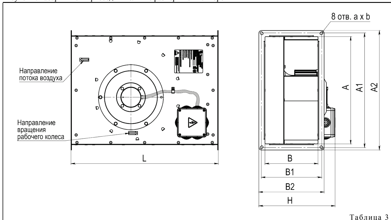
Рисунок 1. Габаритные и присоединительные размеры вентиляторов
