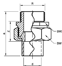
Katalog-Nr. und -bezeichnung 5343g – Verschraubung, konisch dichtend, Lötuffe aus Kupfer, mit Innenlötende, Einschraubteil Außengewinde
