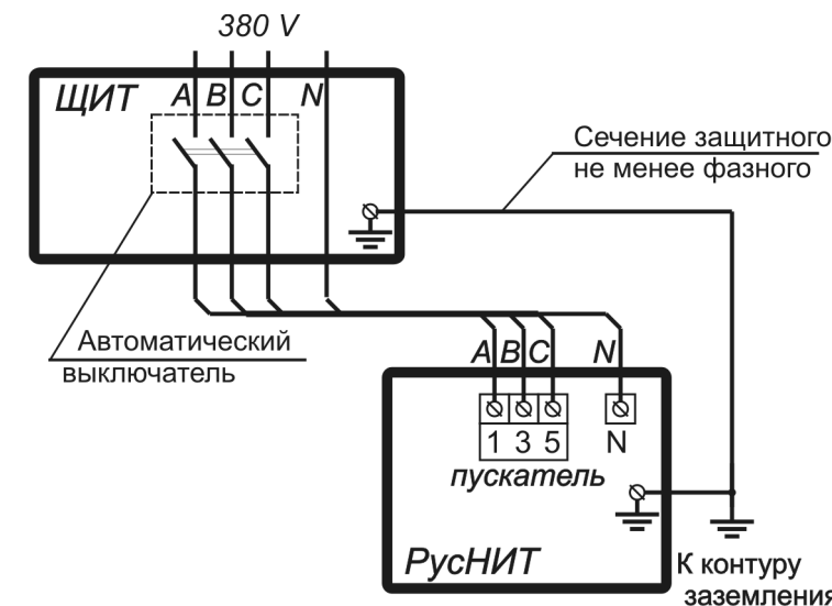
Рис.7. Схема подключения РусНИТ-206НМ, 207НМ, 208НМ, 209НМ к трёхфазной сети.
