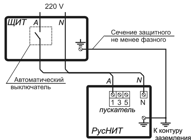
Рис.6. Схема подключения РусНИТ-205НМ,206НМ, 207НМ, 208НМ, 209НМ к однофазной сети .
