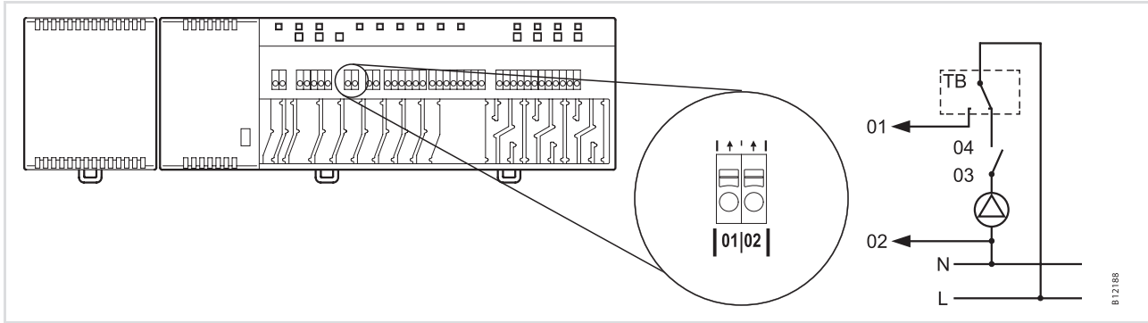
Рис. 28. ТВ-вход как ограничитель температуры
