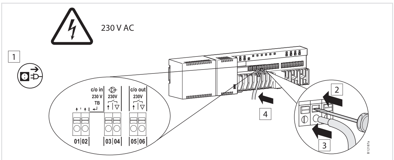
Рис. 22. Подключение проводов
