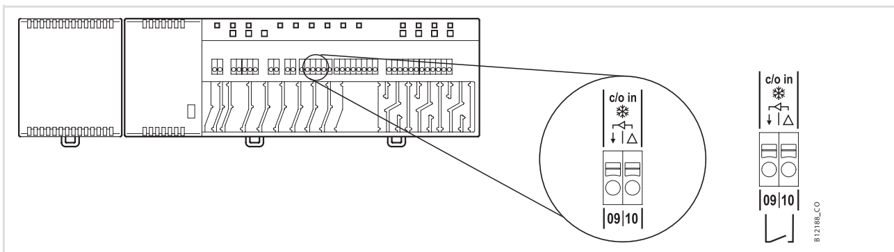
Рис. 29. Переключающий C/O-вход, беспотенциальный контакт
