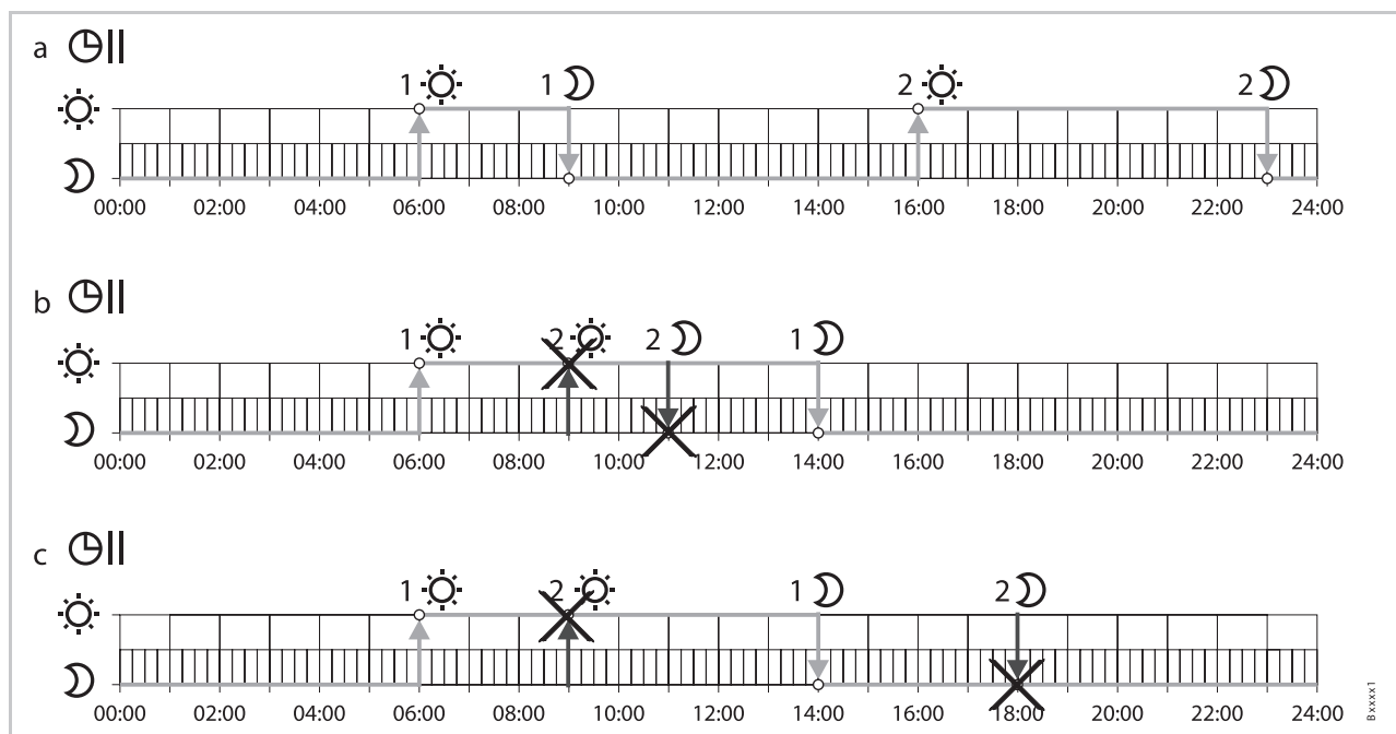
Рис. 36. Правильное и неправильное программирование
