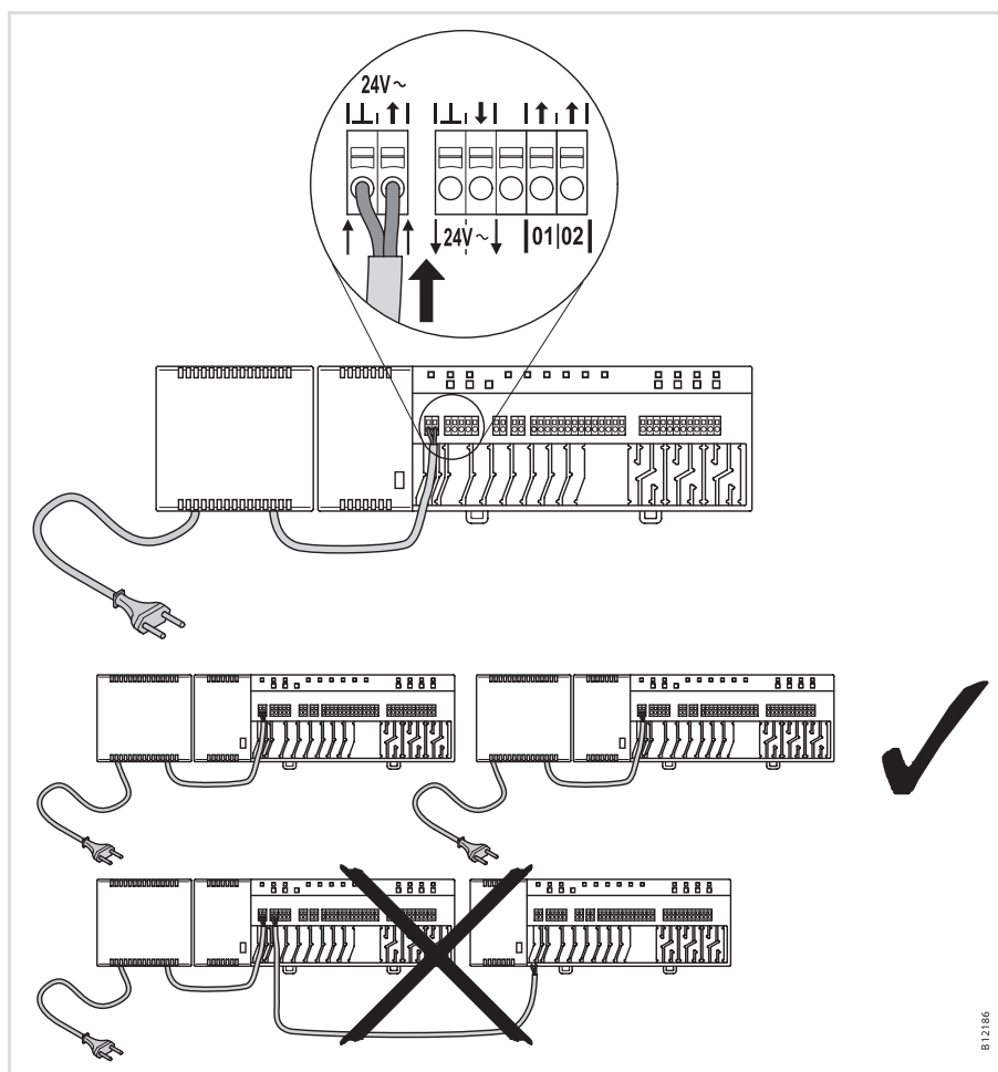
Рис. 21. Подключение трансформатора
