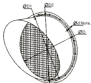
Рисунок 6. Защитный козырек
