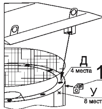
Рисунок 18. Монтаж комплекта крыши
