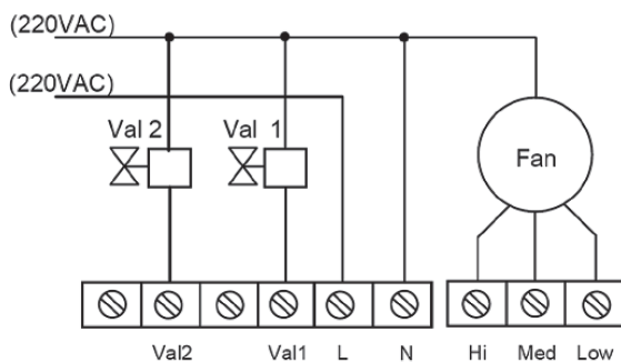
Электрическая схема подключения термостата HR107FCV2
