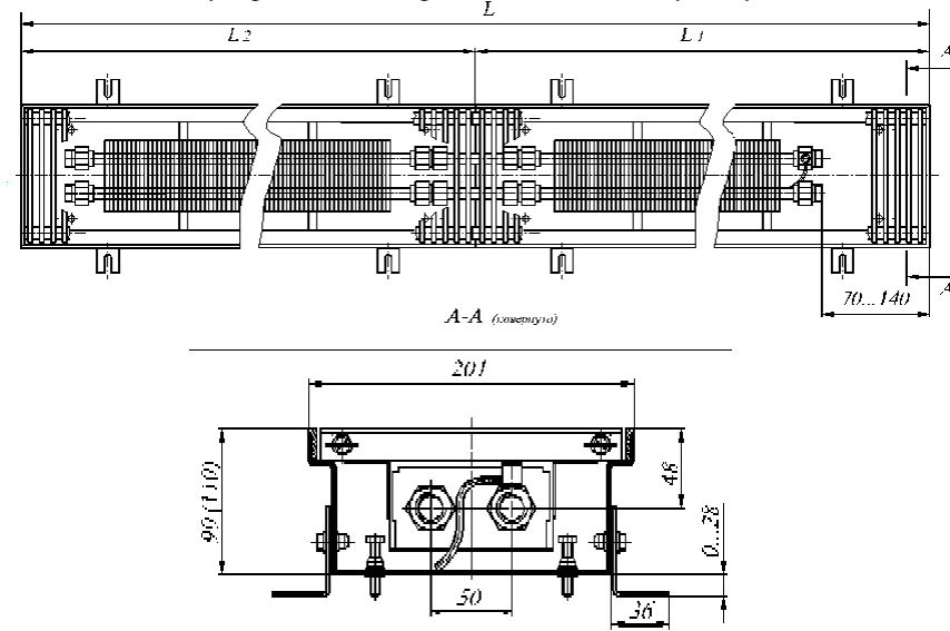
Рис. 1 Конвектор КРК 20.09(11).310...600 концевой 1 - короб установочный; 2 - элемент нагревательный; 3 - решетка; 4 - болты упорные; 5 - опоры; 6 - клапан воздушоспускной;
