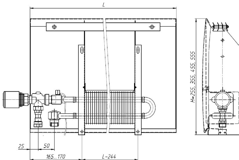
Рис.2 Конвектор настенный с нижним подключением ПКНН – 204...525 А(Р,Р) Т2
