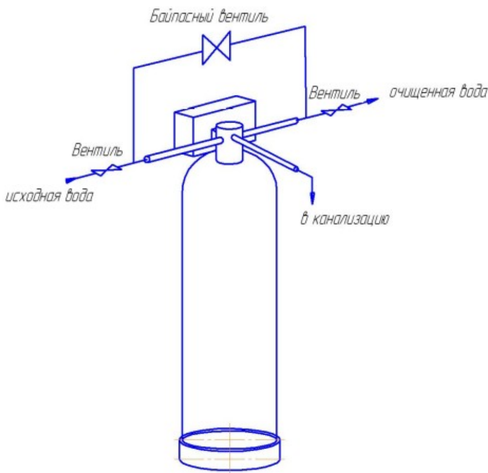
Рисунок 2 — Схема монтажа установки обезжелезивания WFDF-0,7...13,2-Rx-(AC), подключением 3/4", 1", 2".
