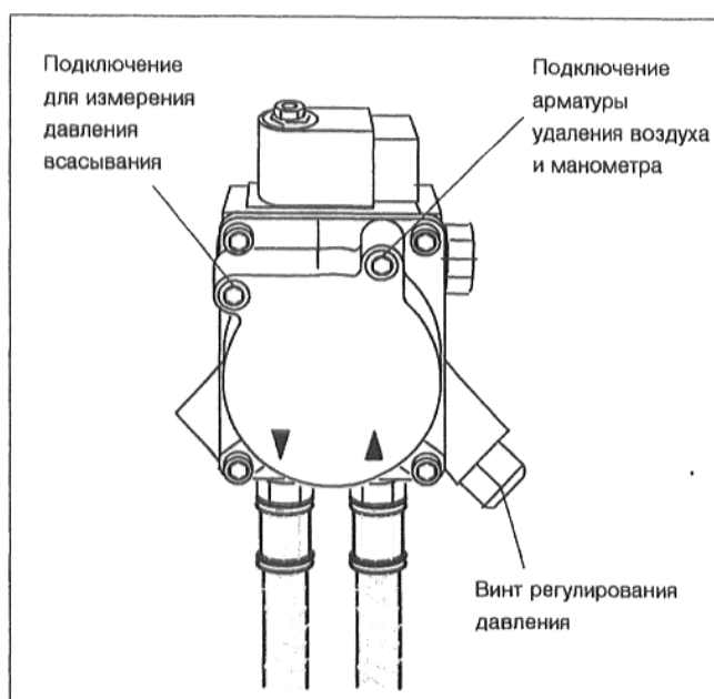
Рис. 1: Насос Suntec типа AL
