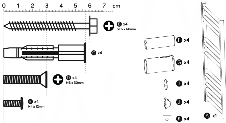
Рисунок 3. Крепежные элементы
