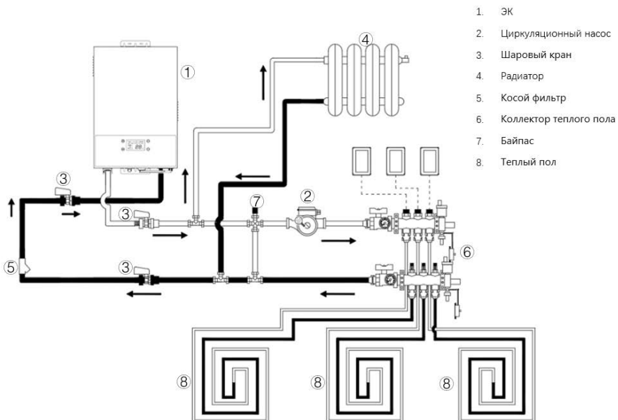
Рис. 8. Схема подключения «теплый пол + ЭК»
