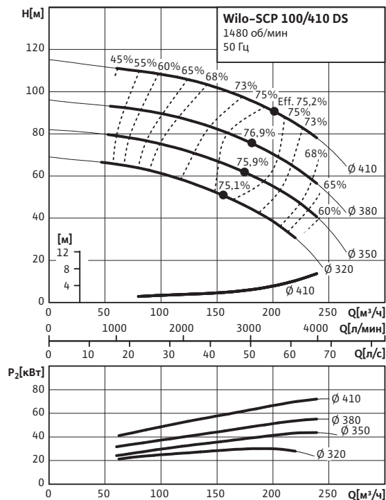
Wilo-SCP 100/410 DS
