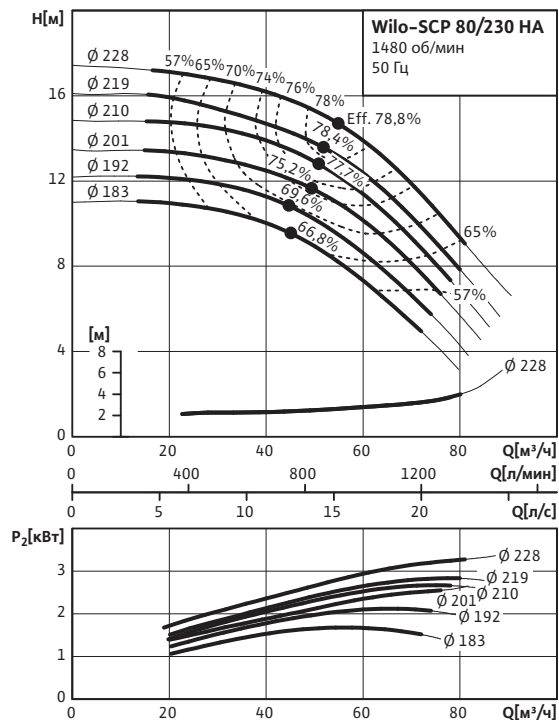
Wilo-SCP 80/230 HA
