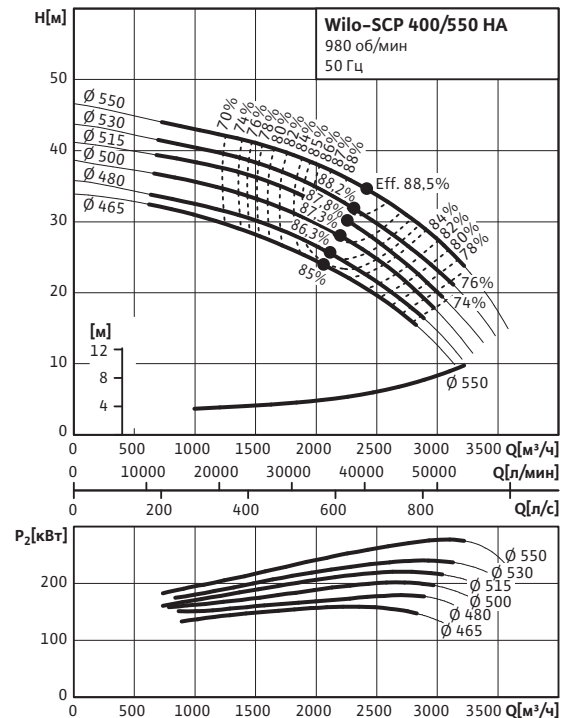
Wilo-SCP 400/550 HA
