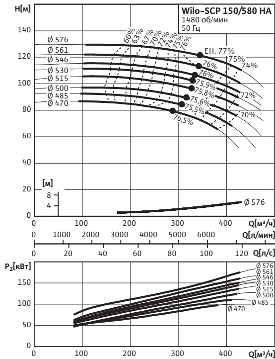
Wilo-SCP 150/580 HA
