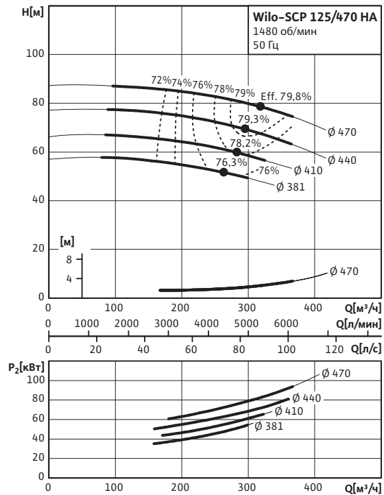
Wilo-SCP 125/470 HA
