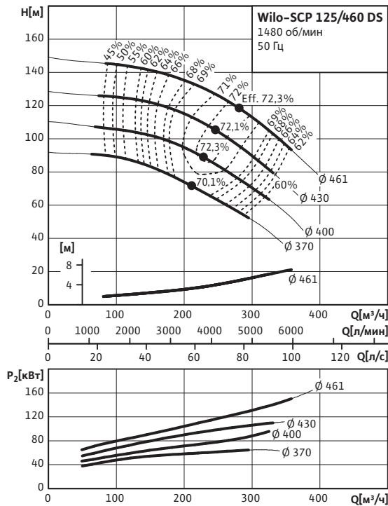
Wilo-SCP 125/460 DS
