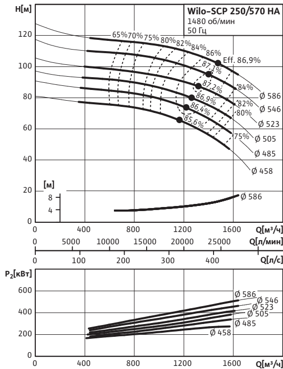
Wilo-SCP 250/570 HA
