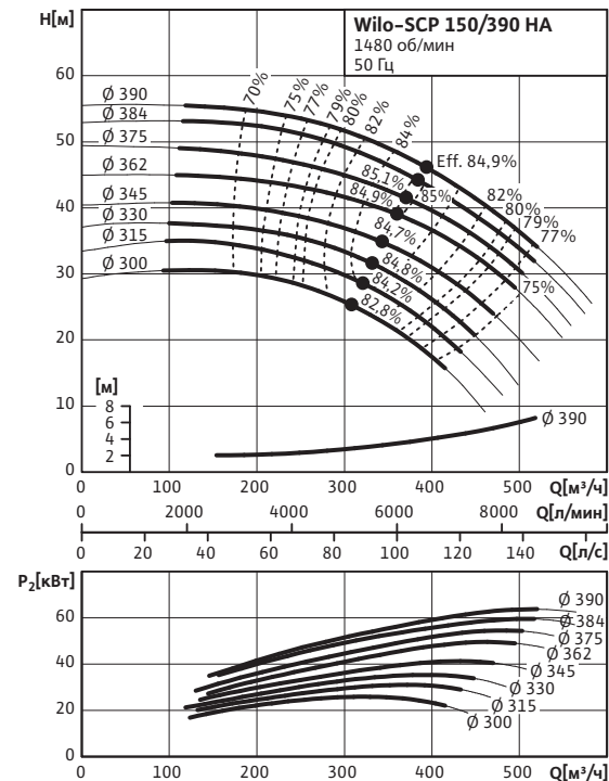
Wilo-SCP 150/390 HA
