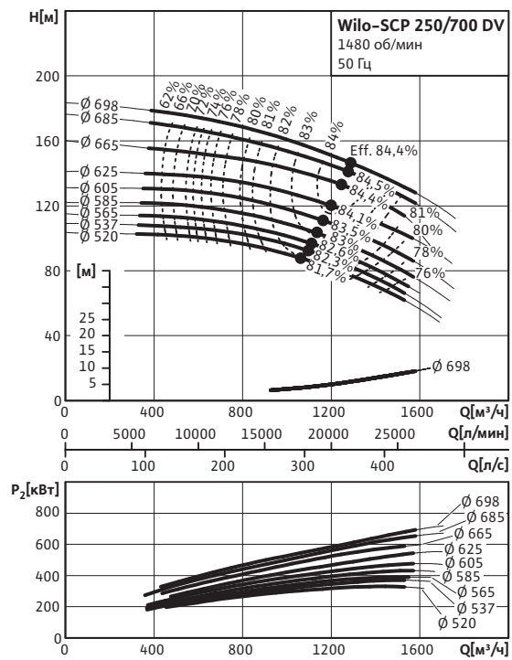
Wilo-SCP 250/700 DV
