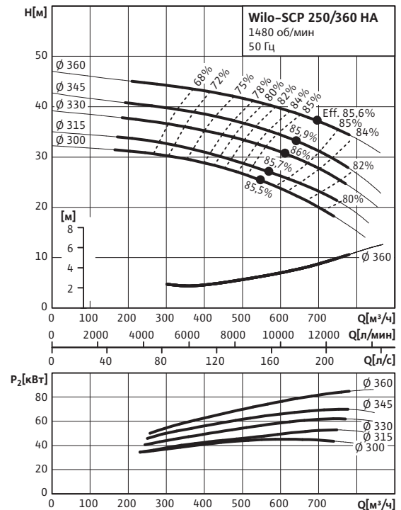
Wilо-SCP 250/360 HA
