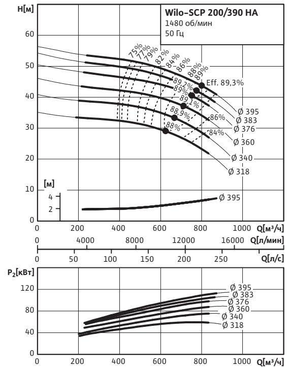
Wilo-SCP 200/390 HA
