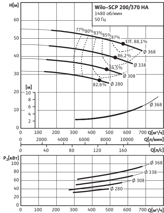
Wilo-SCP 200/370 HA
