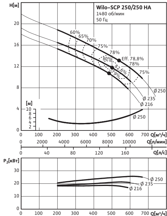
Wilо-SCP 250/250 HA
