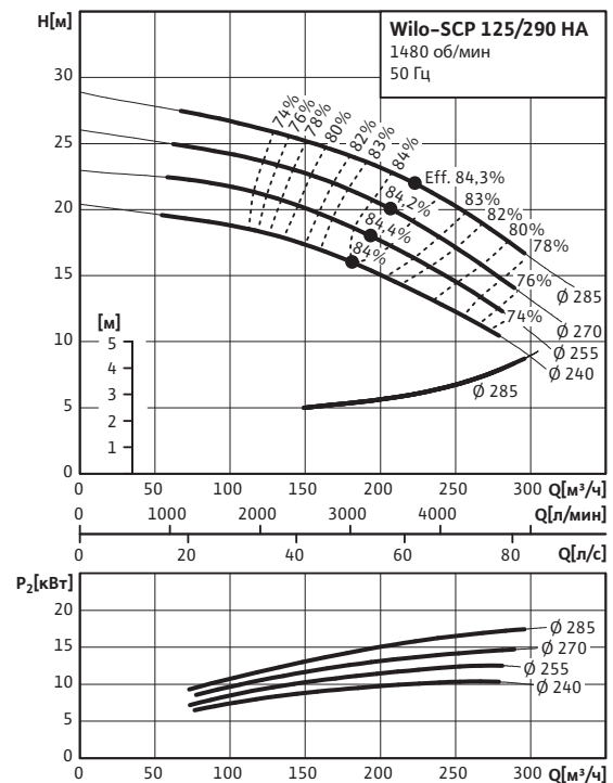
Wilo-SCP 125/290 HA
