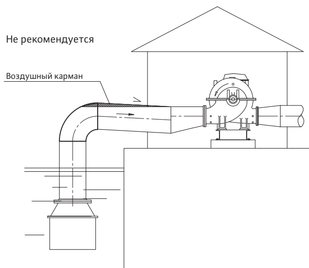
Рис.4. Конструкция всасывающего трубопровода
