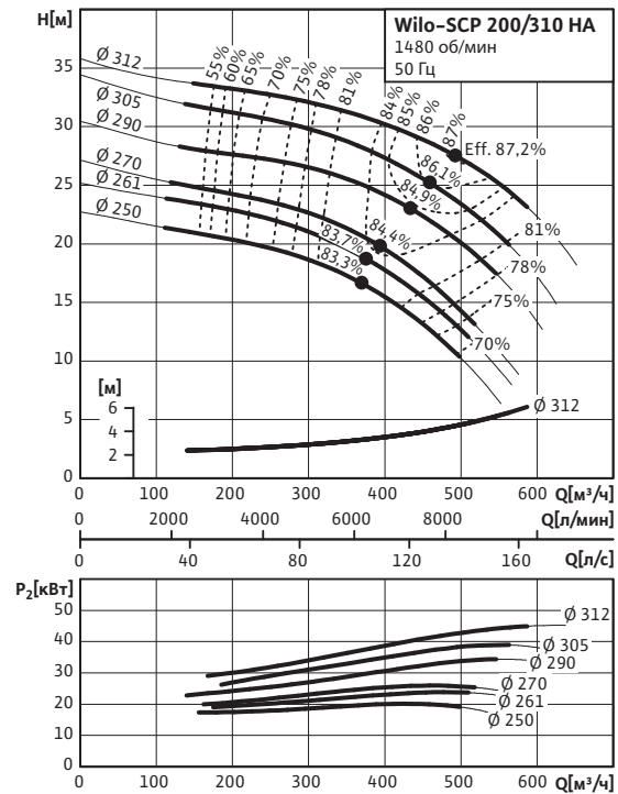
Wilo-SCP 200/310 HA
