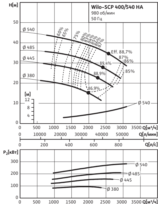
Wilo-SCP 400/540 HA
