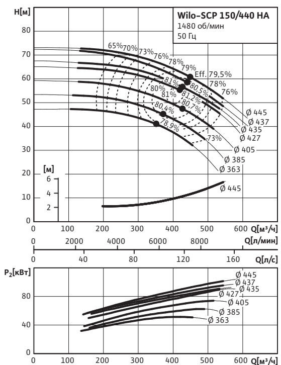
Wilo-SCP 150/440 HA
