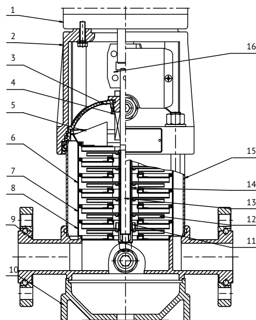
Исполнение с основанием AISI - SBI
