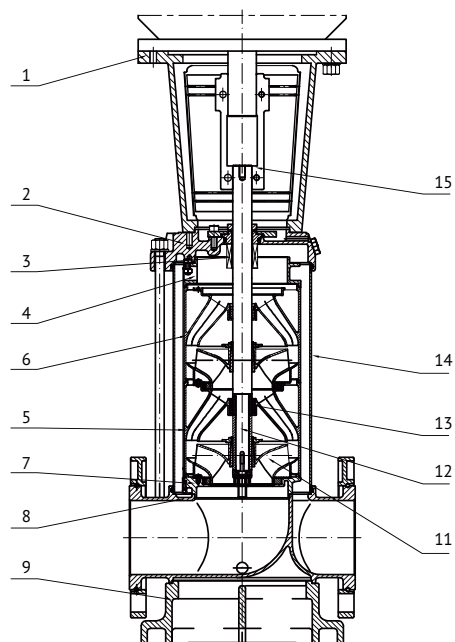
Исполнение с основанием AISI - SBI
