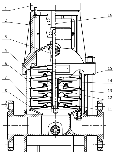
Исполнение стандартное - SB
