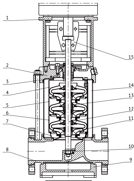
Исполнение с основанием AISI - SBI
