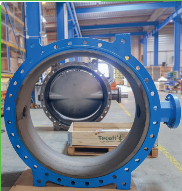
Дисковый поворотный затвор TECWAT Ду1200 Затвор с эпоксидным порошковым покрытием, нанесенным в печи, и затвор перед пескоструйной обработкой
