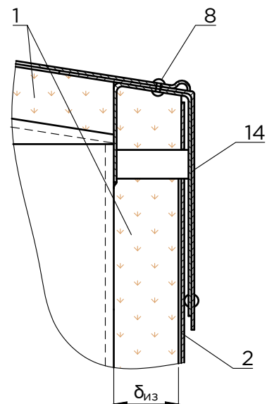
Б - Б
