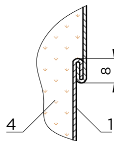
Г - Г
