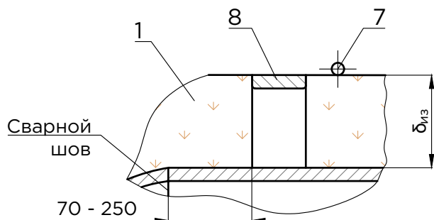
II при изоляции в 1 слой
