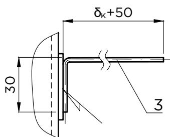
Г - Г
