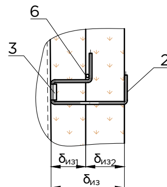
Б - Б вариант
