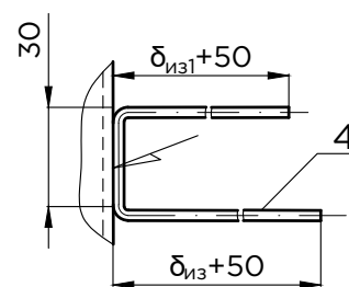
Г - Г
