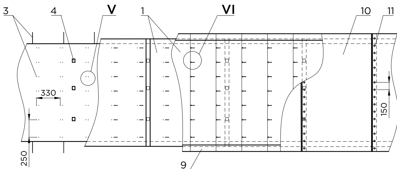
Вид М
