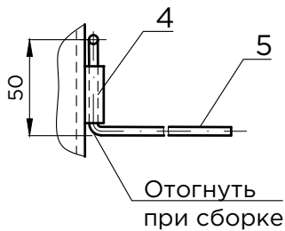
В - В
