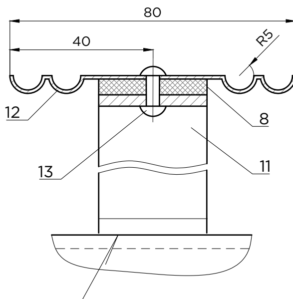
Е - Е
