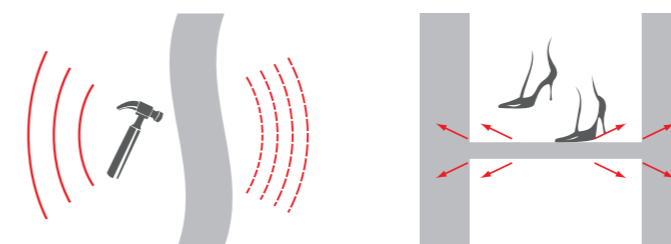
Рисунок 16. Механизм передачи ударного шума
