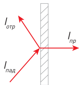
Рисунок 12. Схема прохождения звука через преграду
