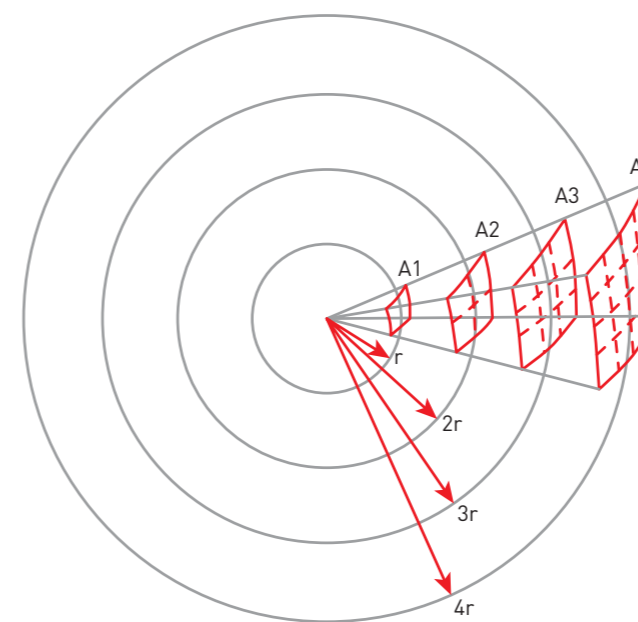
Рисунок 5. Процесс распространения звуковой волны
