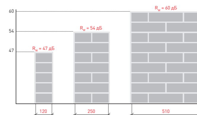
Рисунок 20. Изменение звукоизоляции кирпичной стены при удвоении ее толщины
