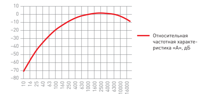
Рисунок 10. Стандартная частотная характеристика «А» шумомера
