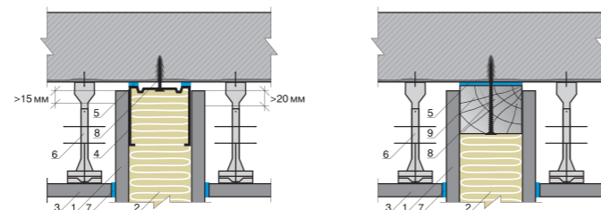
Рисунок 39. Схема примыкания подвесного потолка к перегородке
