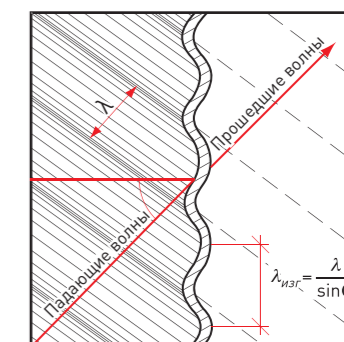
Рисунок 21. Схема возбуждения звуковых колебаний легкой конструкции при косом падении звуковых волн – эффект волнового совпадения
