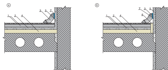
Рисунок 44. Конструктивные решения сопряжений между элементами зданий
