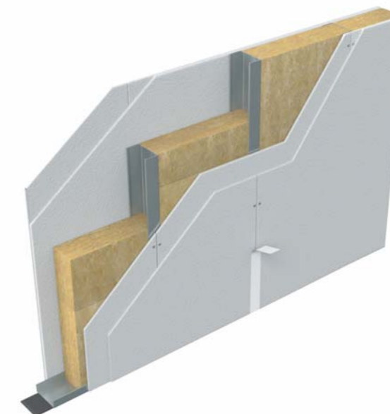
Рисунок 29. Перегородка Тип 3
