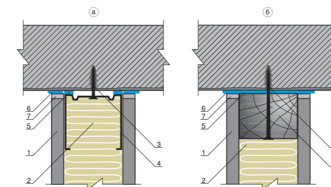
Рисунок 34. Примыкание перегородок к боковым стенам
