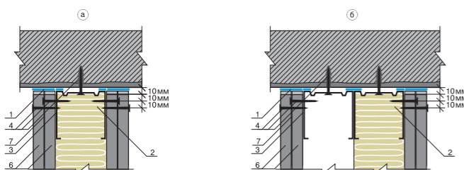
Рисунок 38. Схема крепления двухслойной обшивки из ГКЛ к стойкам каркаса
