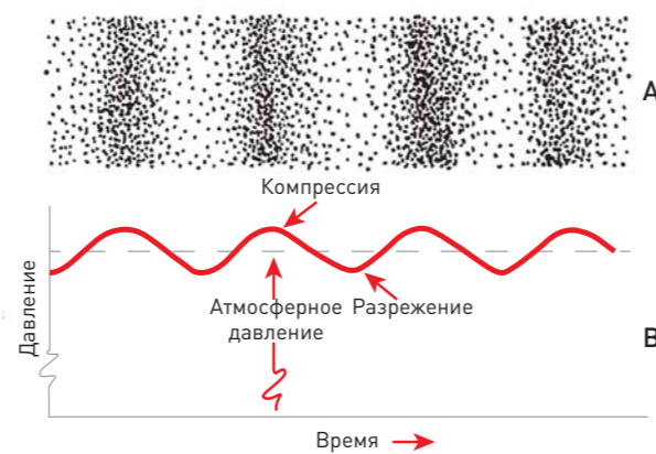
Рисунок 3. Процесс перемещения звуковой волны
