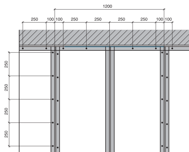
Рисунок 37. Крепление гипсокартонных листов к стойкам каркаса
