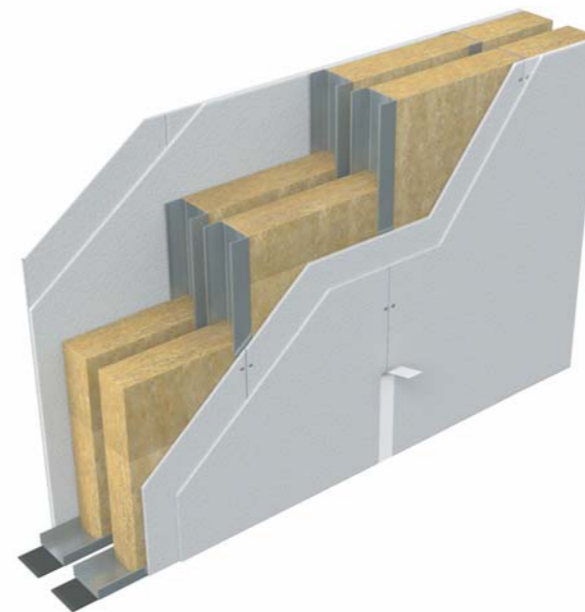
Рисунок 30. Перегородка Тип 4
