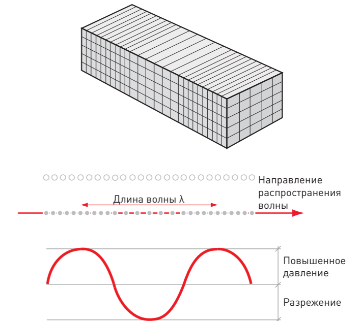
Рисунок 17. Продольная волна. Схема распространения продольной волны в упругой среде
