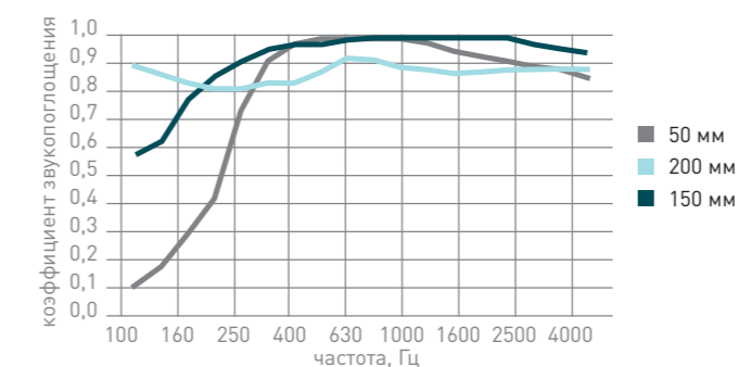
Рисунок 25. Частотные характеристики АКУСТИК БАТТС ПРО
