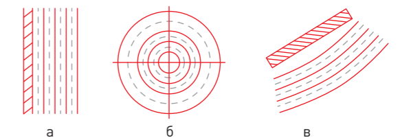
Рисунок 6. Виды источников звука и схематическое изображение фронта волны
