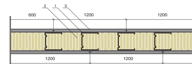
Рисунок 36. Конструктивная схема каркасно-обшивной перегородки
