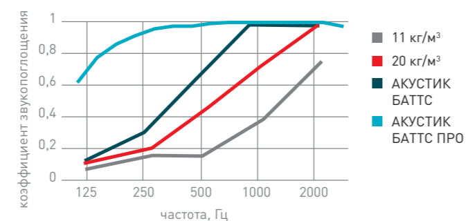
Рисунок 23. Зависимость звукопоглощающих свойств волокнистых материалов от плотности
