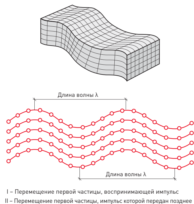
Рисунок 18. Поперечная волна. Схема распространения поперечной волны в упругой среде:
