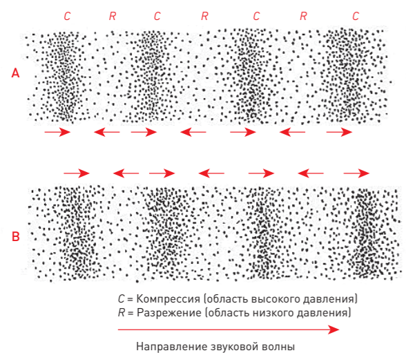
Рисунок 2. Перемещение звуковой волны
