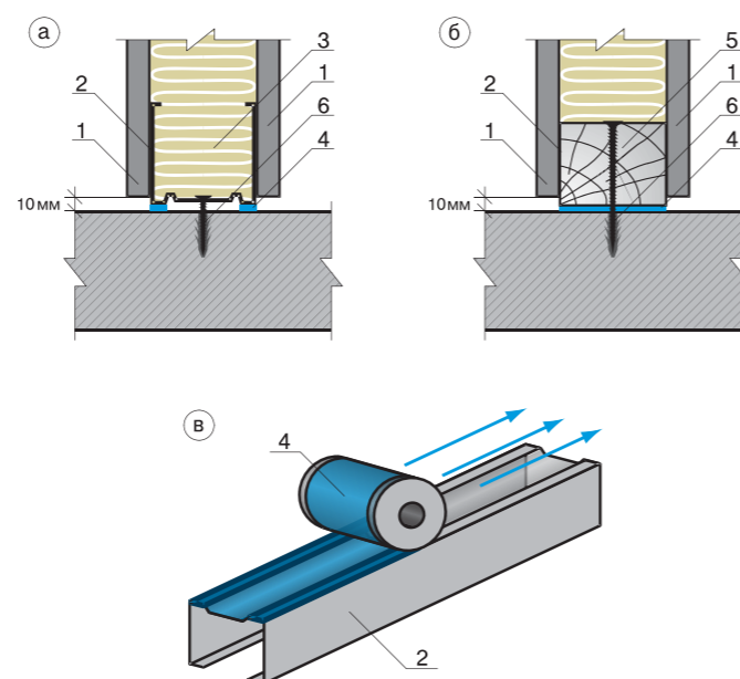
Рисунок 32. Установка перегородки на уплотнительные ленты
