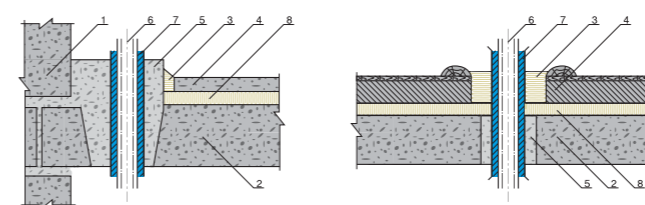
Рисунок 45. Схема пропуска стояка через междуэтажное перекрытие
