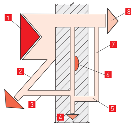
Рисунок 13. Прохождение звука через преграду
