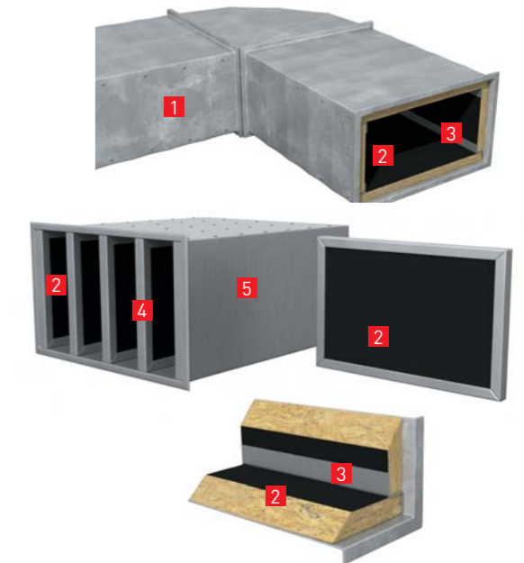
Рисунок 48. Примеры монтажа плит INDUSTRIAL BATTС 80 на воздуховодах
