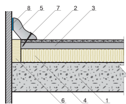
Рисунок 43. Примыкание полов к стенам и перегородкам
