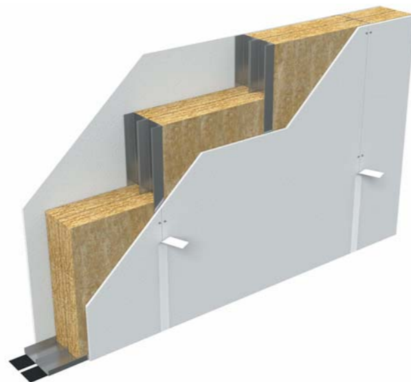
Рисунок 31. Перегородка Тип 5
