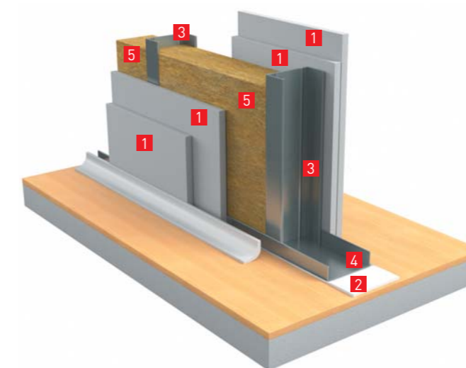
Рисунок 33. Установка перегородки на основание пола
