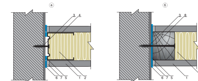
Рисунок 35. Примыкание перегородок к боковым стенам
