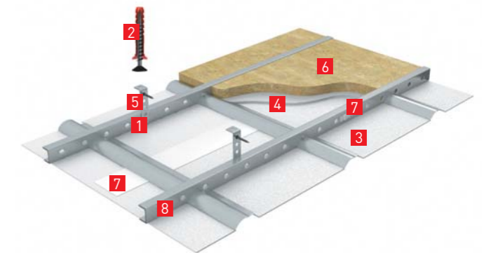
Рисунок 46. Конструктивная схема подвесного потолка
