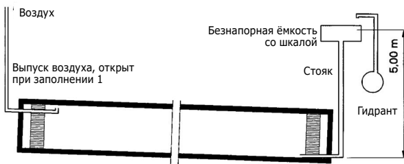
Рис. 10 Проверка герметичности
